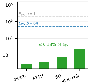
(d) hand-off energy by bearer
