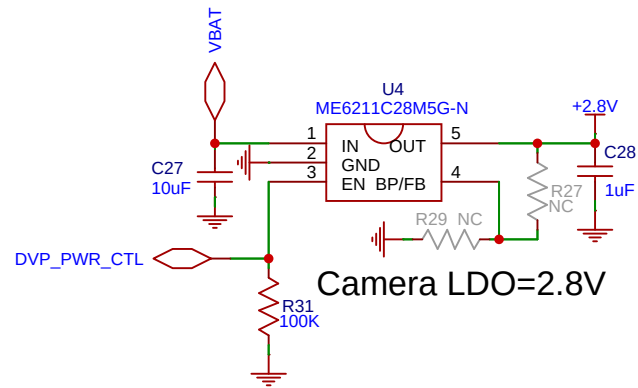
外部LDO
