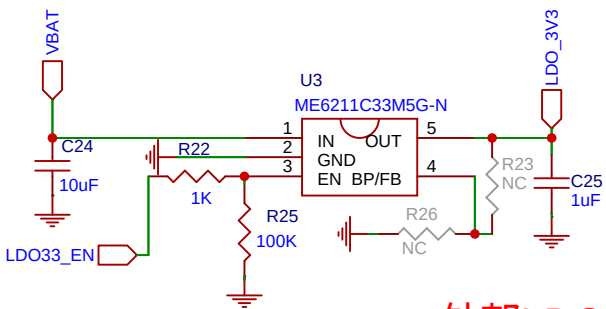
外部LDO
