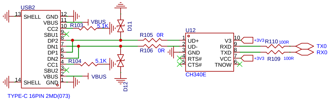
USB
