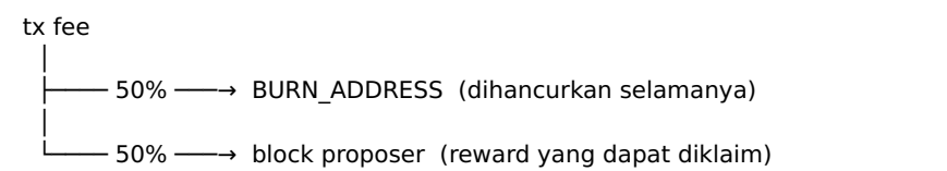
Gambar 3 — Aliran pembagian fee
