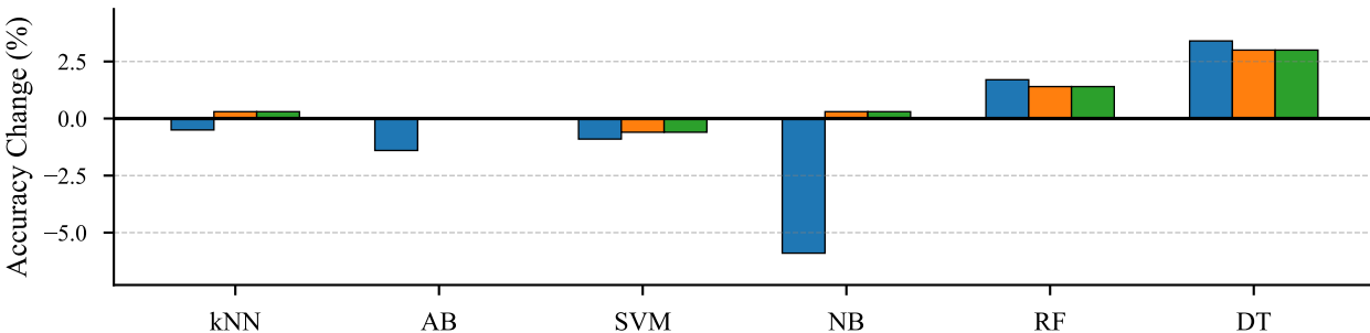
WDBC Dataset
