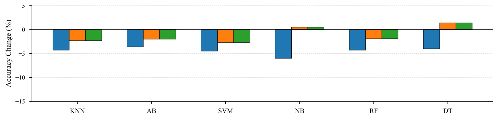
WDBC Dataset
