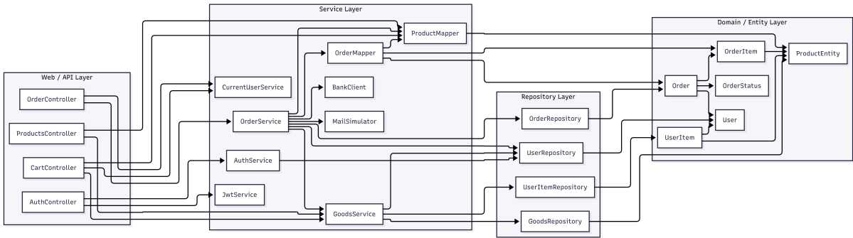
Рисунок 2: UML-диаграмма классов
