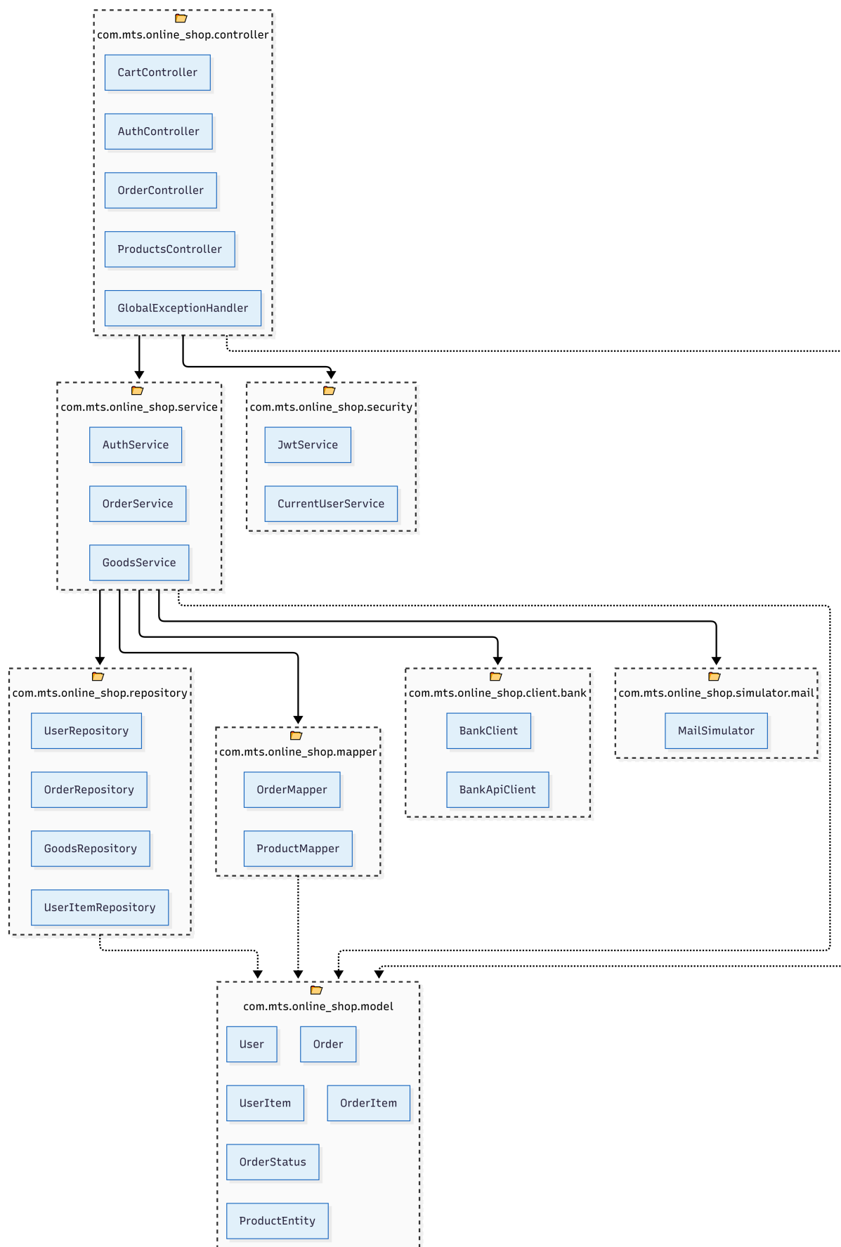
Рисунок 3: UML-диаграмма пакетов
