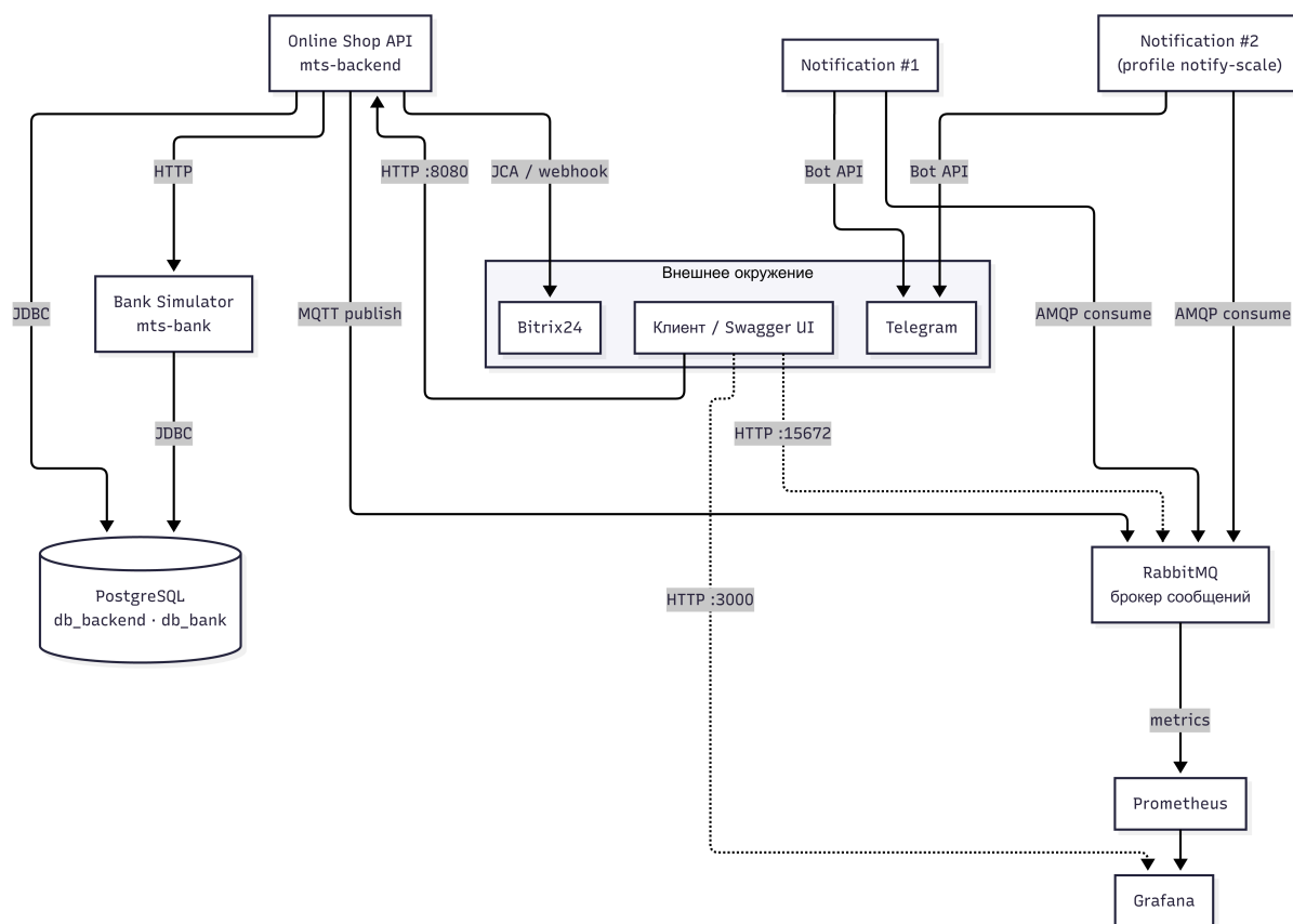
Рисунок 4: UML-диаграмма развертывания
