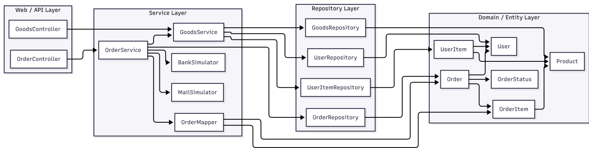
Рисунок 2: UML-диаграмма классов
