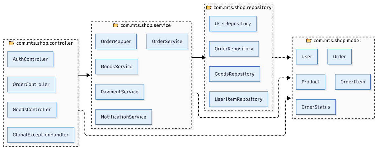
Рисунок 3: UML-диаграмма пакетов
