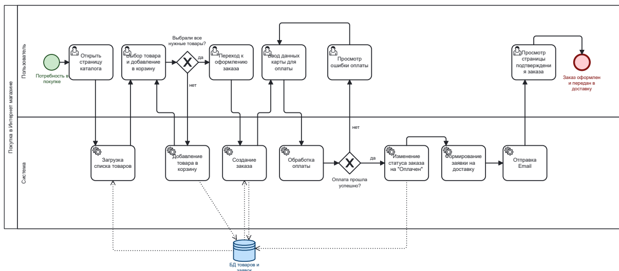
Рисунок 1: BPMN диаграмма
