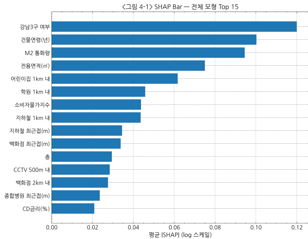
<그림 4-1> SHAP Bar — 전체 모형 상위 15 변수
