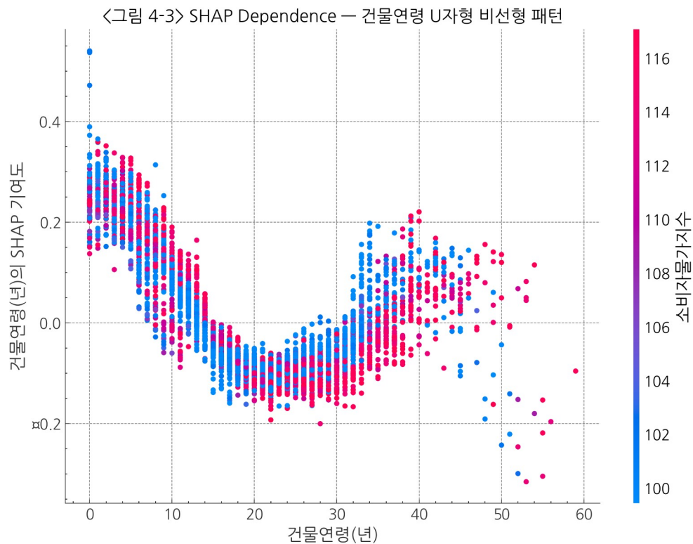
〈그림 4-3〉 건물연령 SHAP Dependence — U자형
