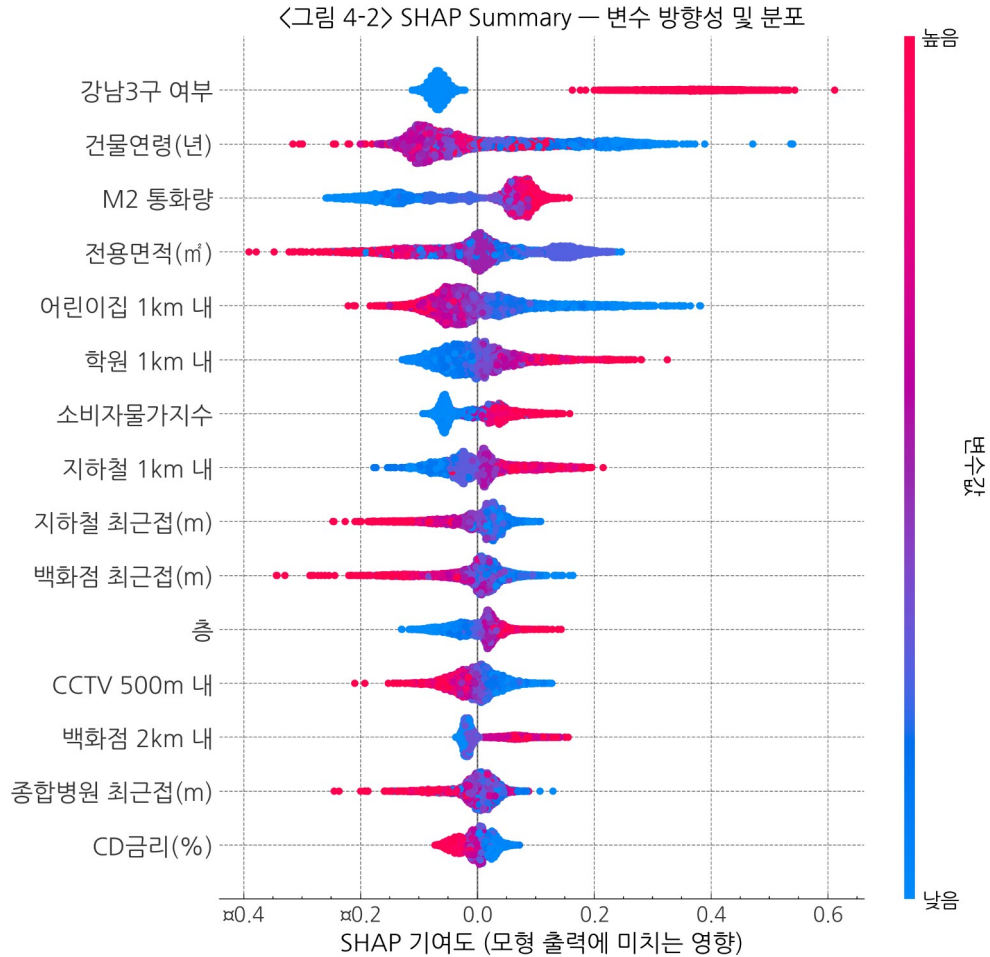
<그림 4-2> SHAP Summary — 변수 방향성 및 분포
