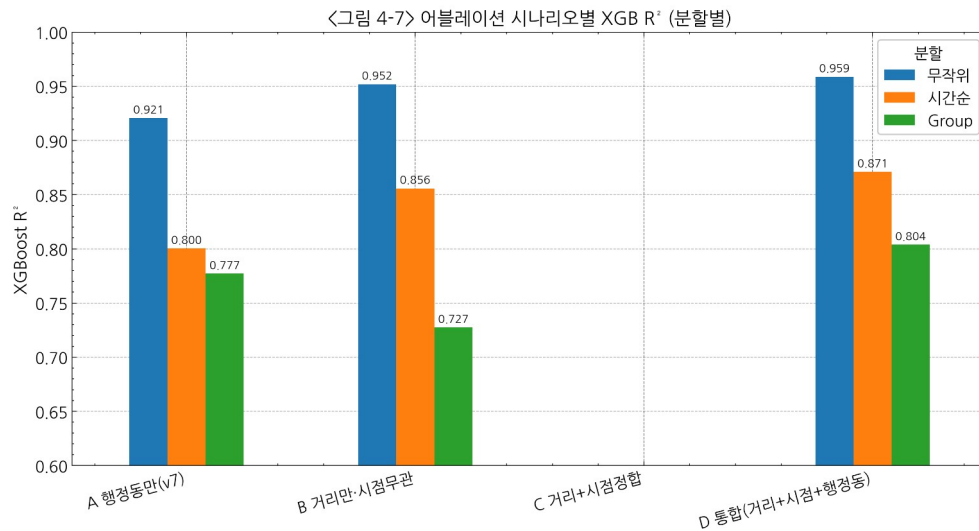
<그림 4-7> 어블레이션 시나리오별 XGB R^2
