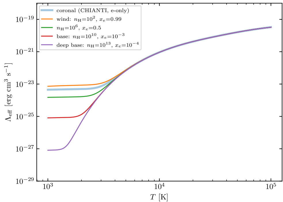
O I
