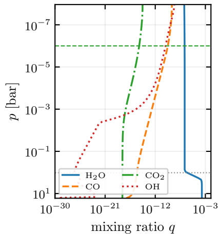
(d) the column, by reservoir
