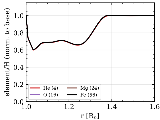
element diffusion (v2)
