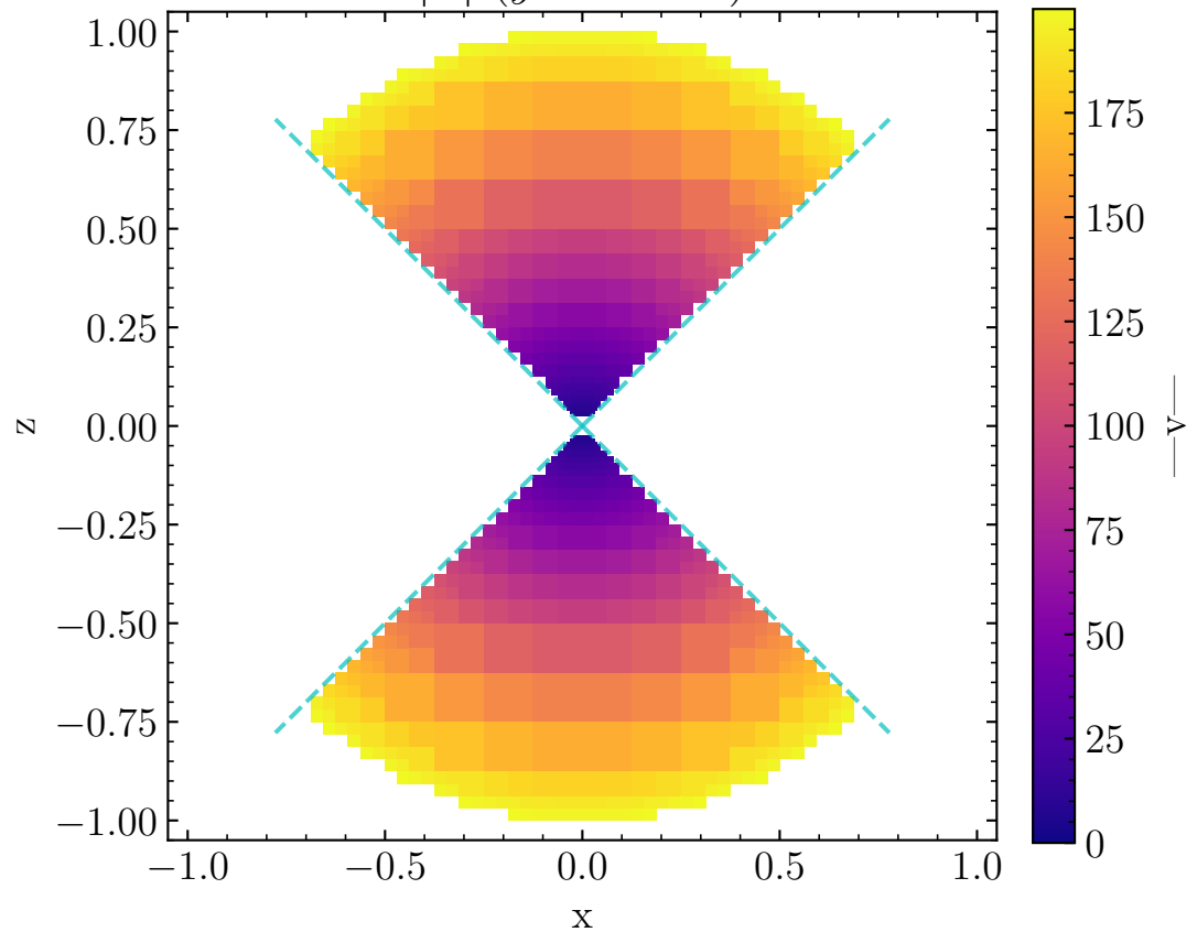
|\mathbf{v}| ( y = 0 slice)
