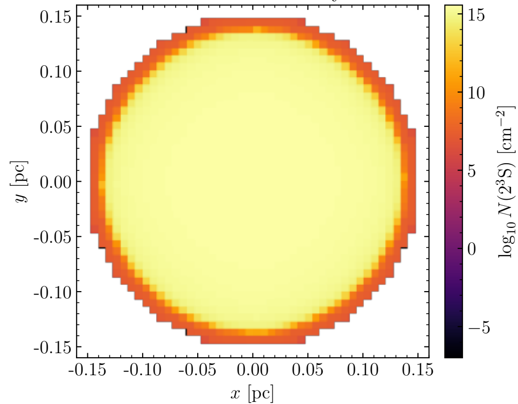
2^3\text{S} column density
