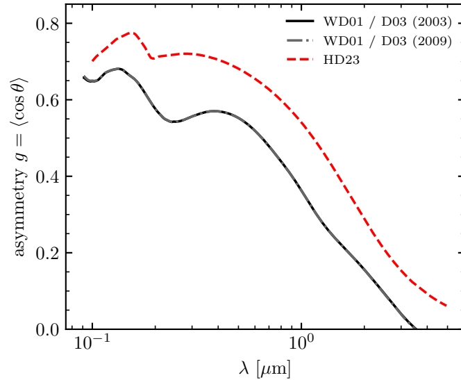
Asymmetry parameter
