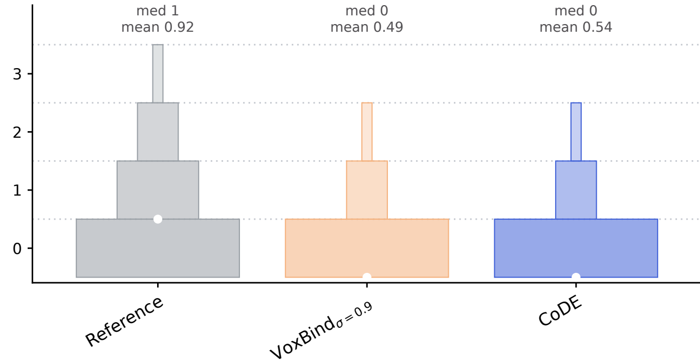
H-bonds donor
