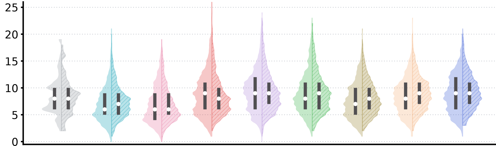
van der Waals contacts
