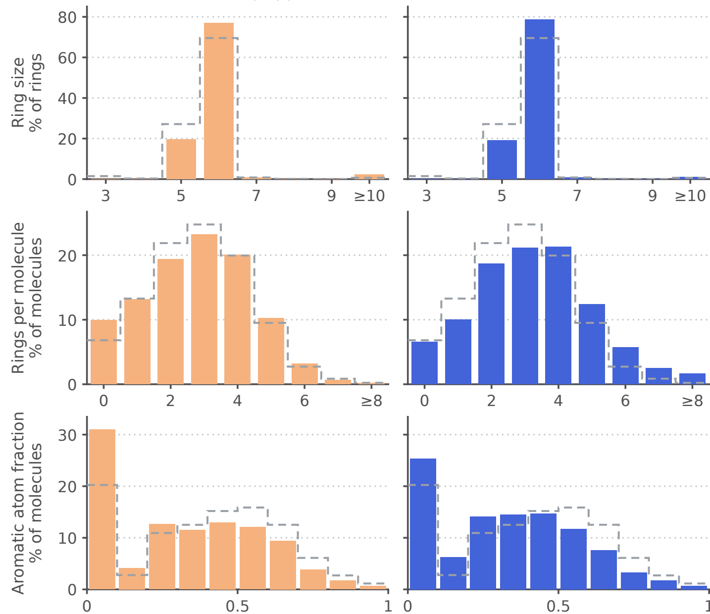
VoxBind _{\sigma=0.9}
