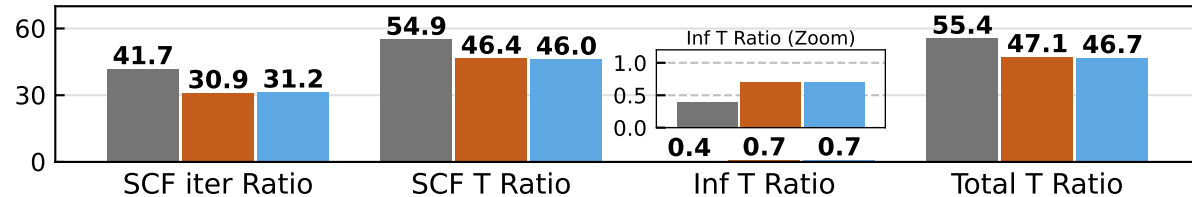
QH9-dynamic (300k-mol)
