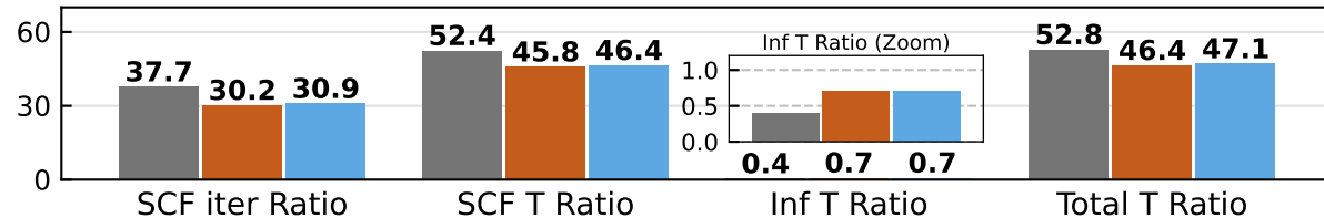
QH9-stable (ood)
