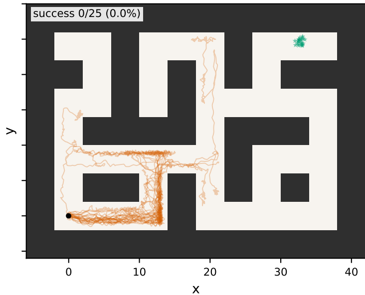
TD3+RAPO
