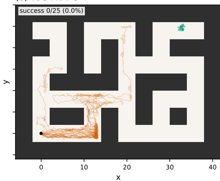
(b) TD3+RAPO
