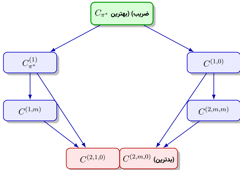
جدول ۸۹: مقایسه مشخصه‌های نظری الگوریتم‌های تکرار خطمشی تقریبی [۴۸۸]
