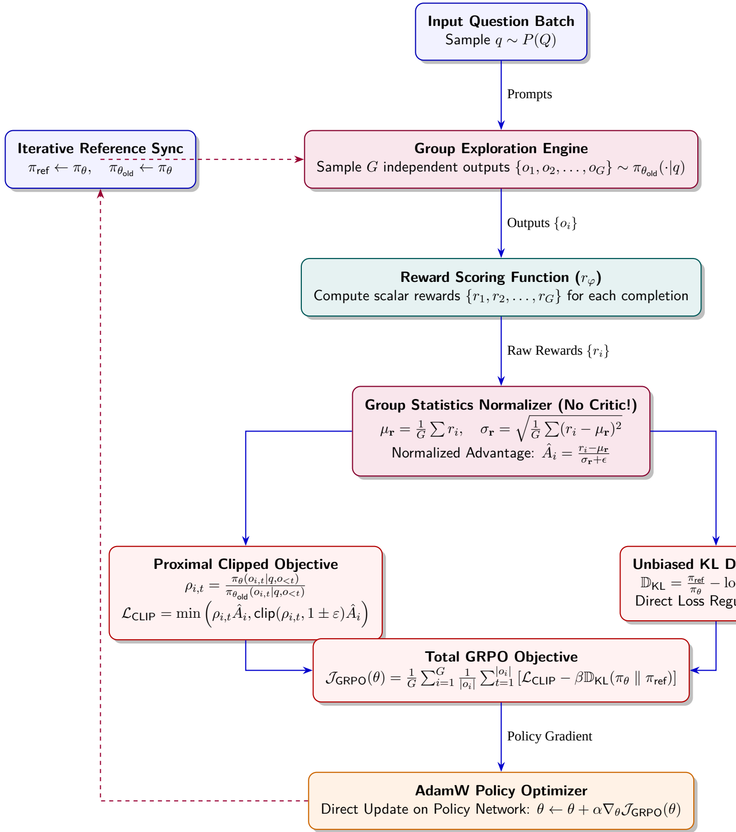
شکل ۸: دیاگرام جامع جریان داده‌ها، ارزیابی آماری گروهی و به‌روزرسانی بدون منتقد در الگوریتم GRPO.
