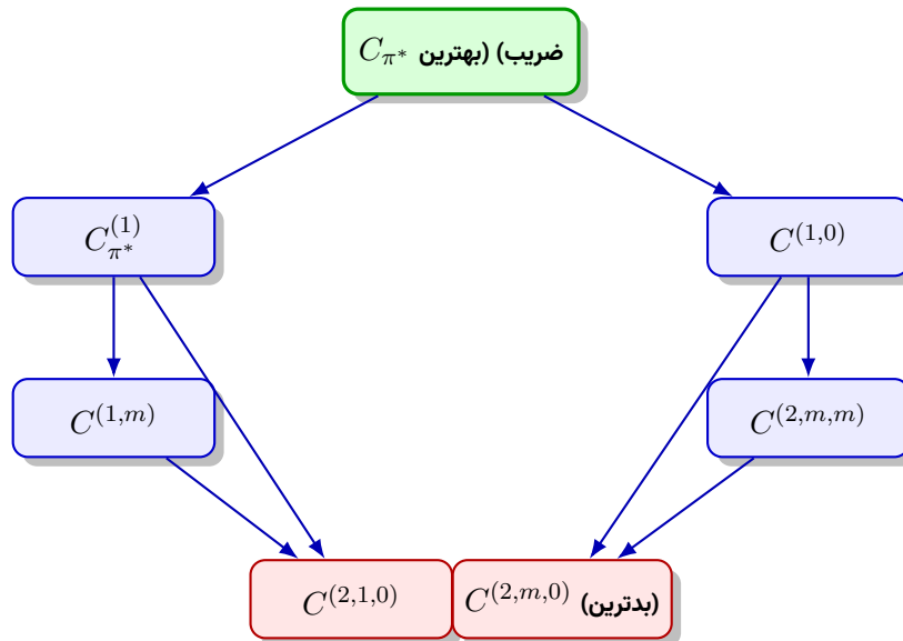
جدول ۵۸: مقایسه مشخصه‌های نظری الگوریتم‌های تکرار خط‌مشی تقریبی [۲۳۷]
