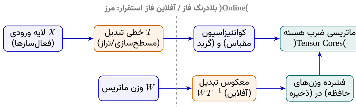
شکل ۸۳: جریان پردازش داده در خط لوله کوانتیزاسیون مدرن مدل‌های زبانی بزرگ.
