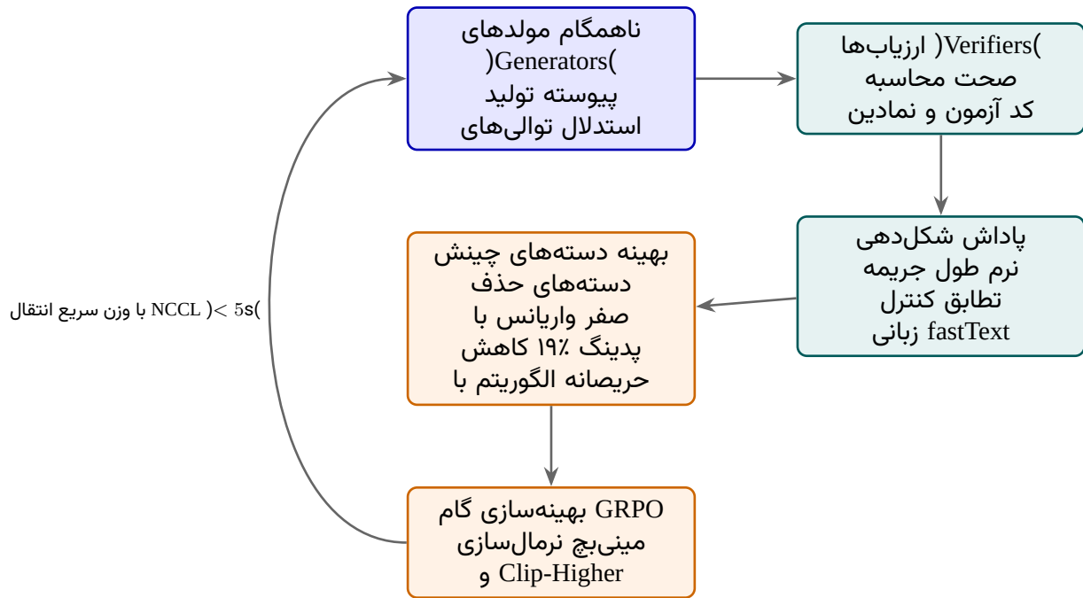
شکل ۷۷: پایپ‌لاین بهینه‌سازی نهمگام مدل Magistral
