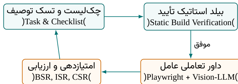
شکل ۹۴: چرخه بسته ارزیابی Agent-as-a-Judge در ارزیابی فرانت‌اند GLM-5
