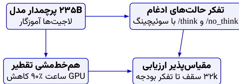
شکل ۹۹: جریان تقطیر و ارزیابی حالات پاسخ‌دهی در مدل‌های Qwen3
