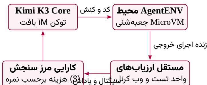
شکل ۹۵: چارچوب ارزیابی جعبه‌شنی و سنجش کارایی هزینه در Kimi K3
