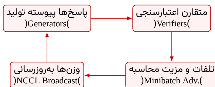
شکل ۹۶: خط لوله بازخورد بلادرنگ در ارزیابی مدل Magistral
