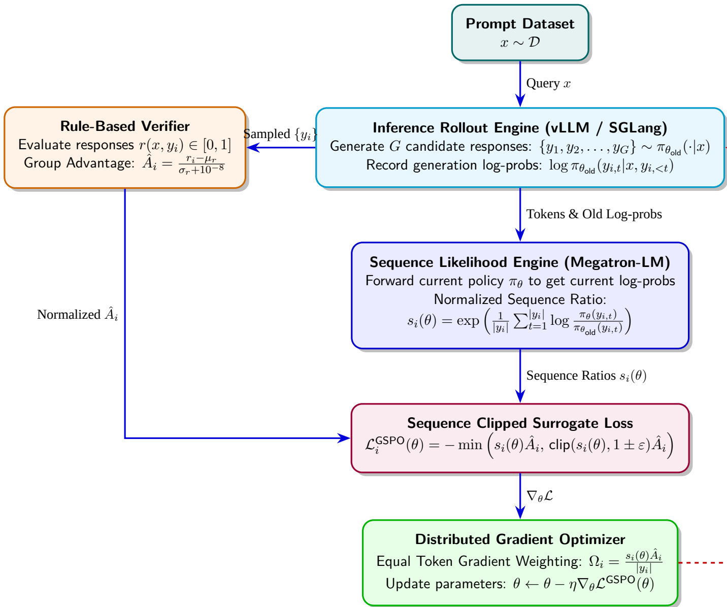
شکل ۱۰۳: دیاگرام جامع معماری خط لوله آموزش، محاسبه نسبت اهمیت توالی با نرمال‌سازی طولی و به‌روزرسانی گرادین همگن در الگوریتم GSPO.
