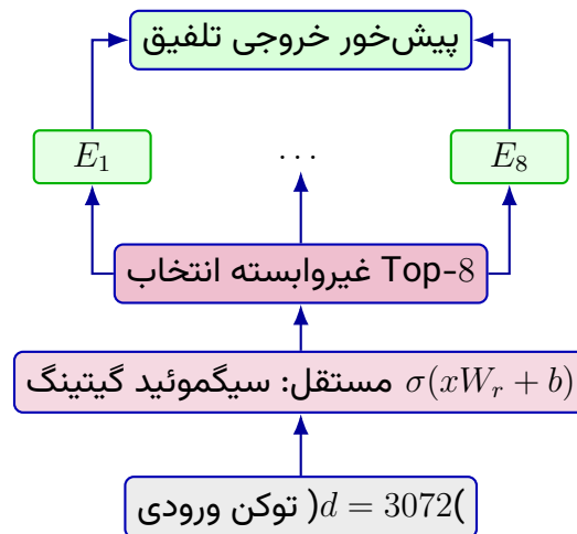
شکل ۲۷: مکانیزم گیتینگ سیگموئیدی مستقل در لایه‌های MoE مدل MiniMax-M2.
