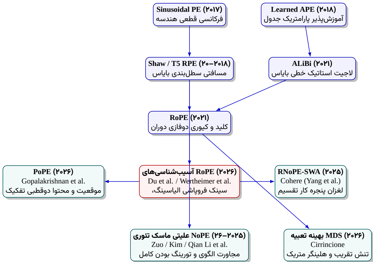
شکل ۱۳: تبارشناسی، سیر تکاملی و الگوهای ساختاری روش های کدگذاری موقعیت در مدل های ترنسفورمر
