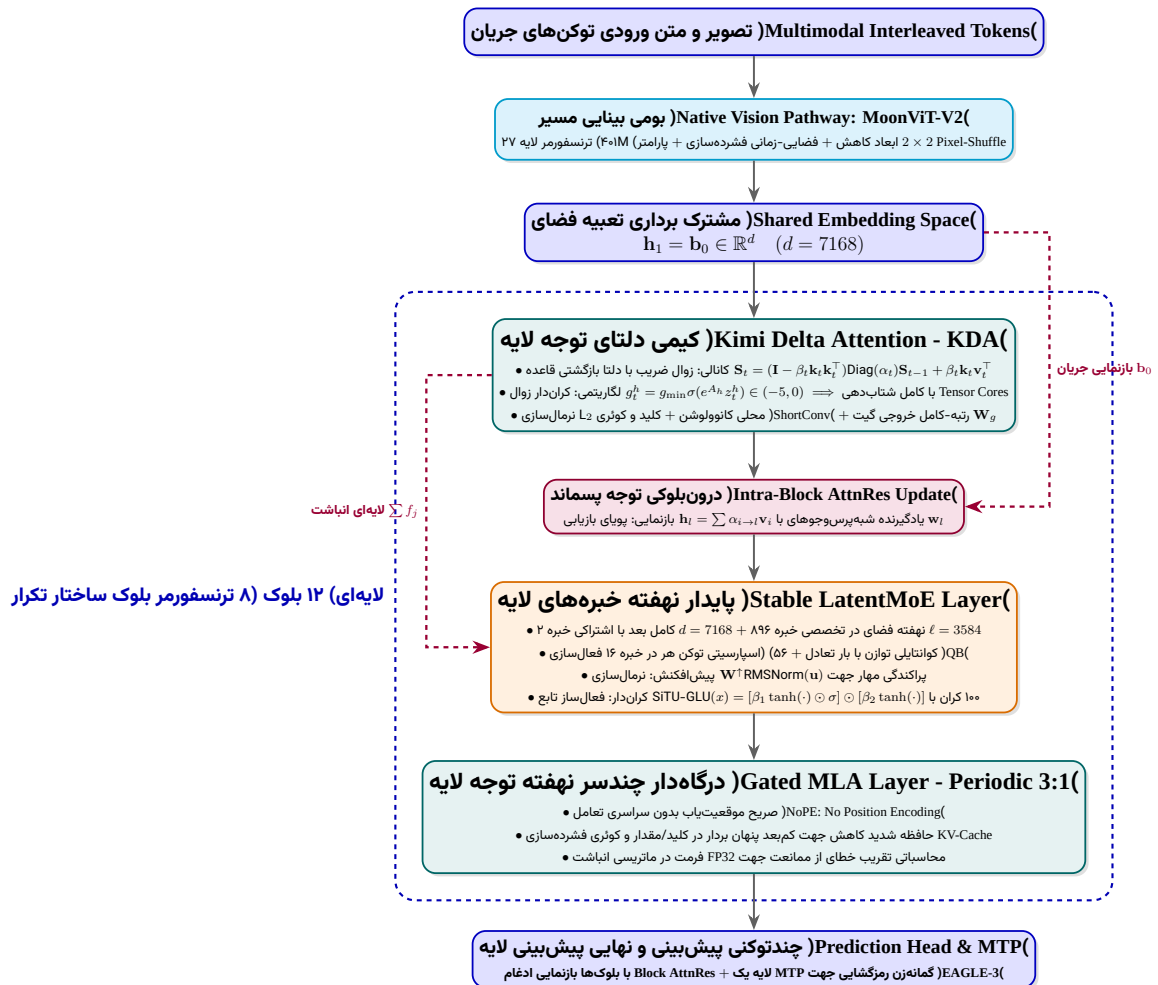
شکل ۴۵: معماری یکپارچه بلوک ترنسفورمر Kimi K3 شامل توجه هیبریدی، Stable و Block AttnRes، LatentMoE.
