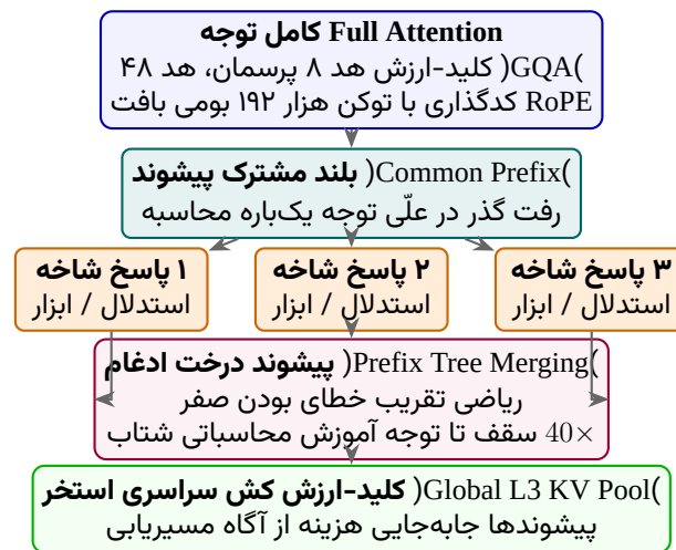
شکل ۵۹: معماری توجه کامل و شتاب‌دهی ساختار کش از طریق ادغام درخت پیشوند در MiniMax-M2.
