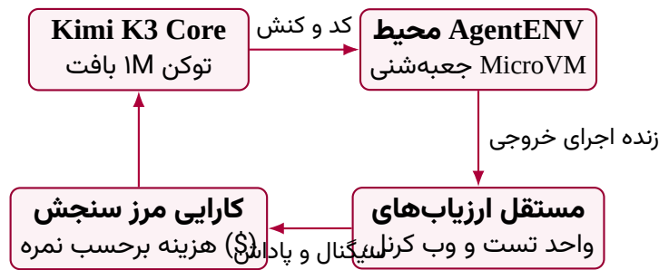
شکل ۱۰۶: چارچوب ارزیابی جعبه‌شنی و سنجش کارایی هزینه در Kimi K3
