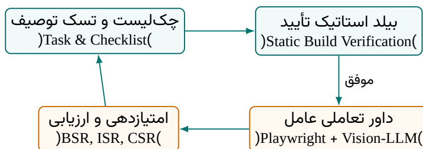
شکل ۱۰۵: چرخه بسته ارزیابی Agent-as-a-Judge در ارزیابی فرانت‌اند GLM-5
