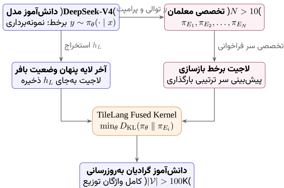
شکل ۹۴: سازوکار تقطیر برخط چندمعلمی با بازسازی بلادرنگ لاجیت در DeepSeek-V4
