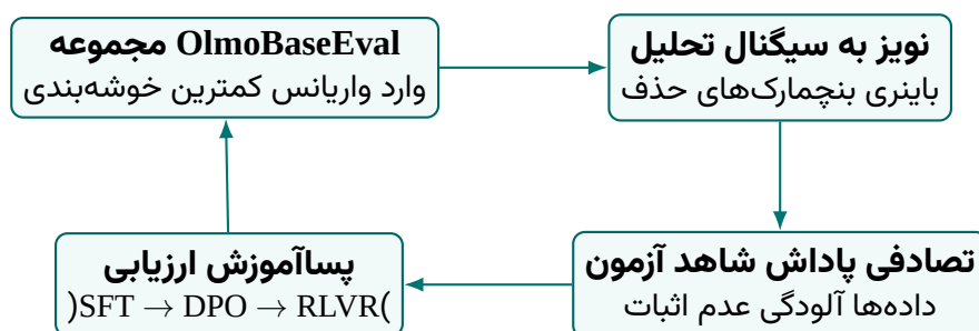
شکل ۱۱۱: چارچوب پایش کیفیت و عدم آلودگی داده‌ها در ارزیابی OLMo 3
