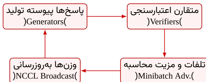
شکل ۱۰۷: خط لوله بازخورد بلادرنگ در ارزیابی مدل Magistral
