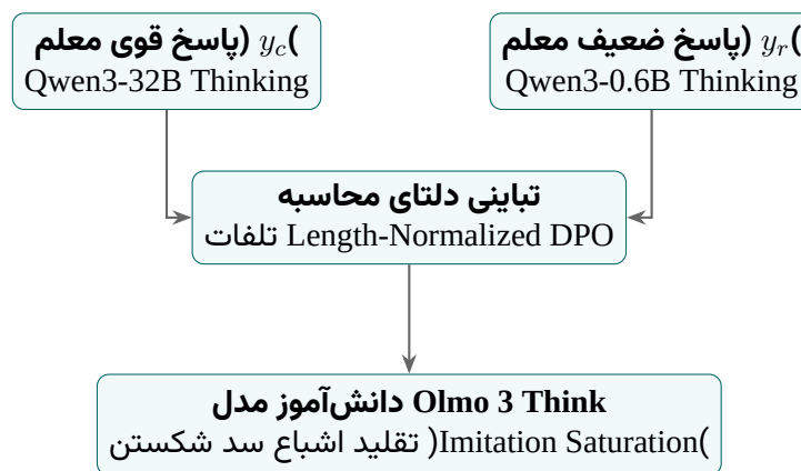
شکل ۱۰۱: سازوکار یادگیری دلتا (Delta Learning) در برابر اشباع تقلید در Olmo 3
