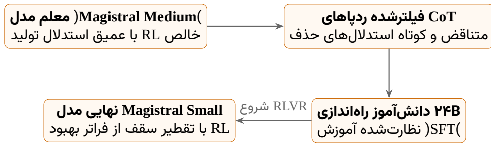
شکل ۹۷: فرایند تقطیر و ارتقای متوالی در Magistral Small
