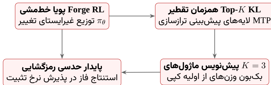
شکل ۹۸: تقطیر همزمان لایه‌های MTP با استفاده از Top-K KL در MiniMax-M2
