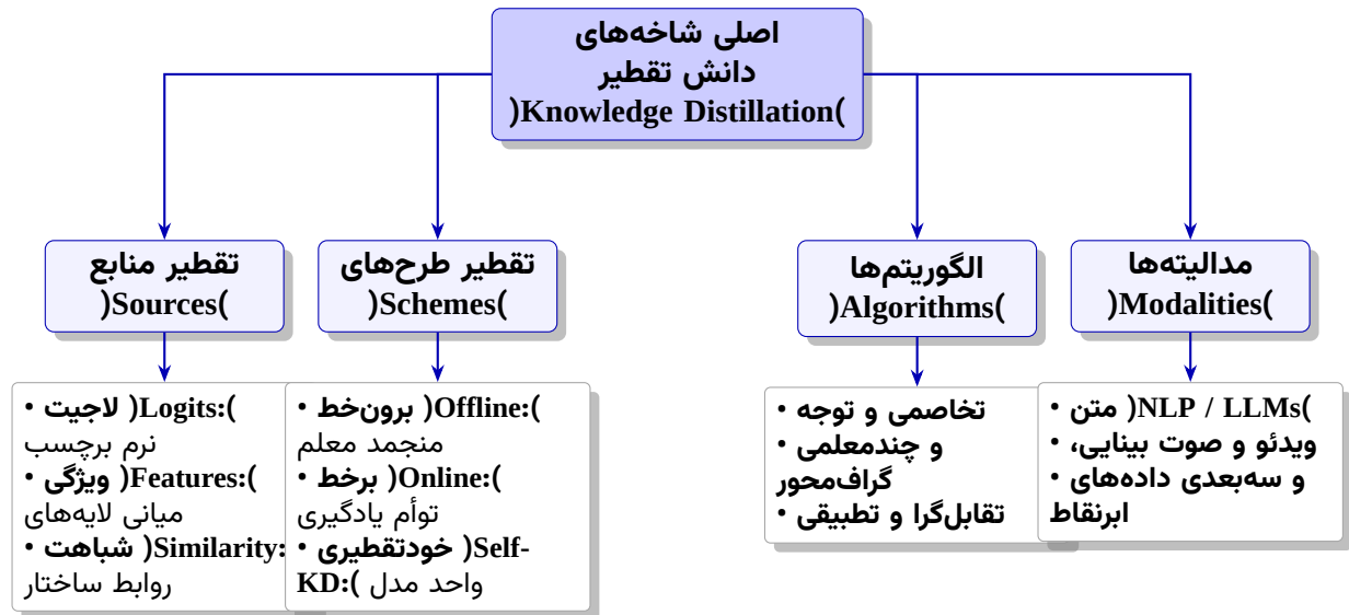
شکل ۹۳: درخت ساختاریافته ابعاد گوناگون تقطیر دانش بر پایه گونه‌شناسی منصورین و همکاران [۵۳۴].
