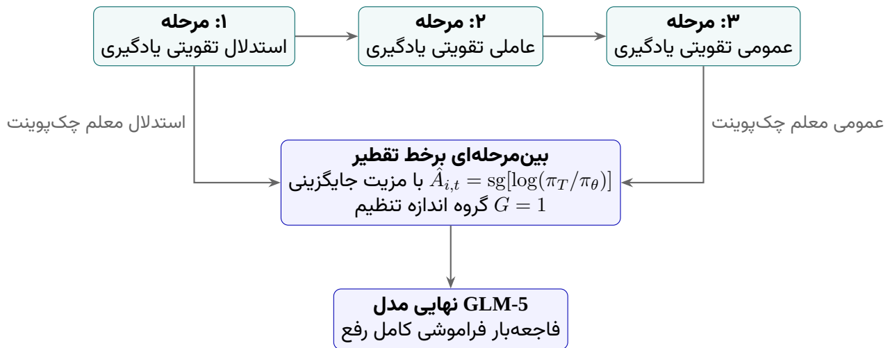
شکل ۹۵: خطلوله تقطیر برخط بین مرحله ای در GLM-5 برای بازیابی مهارت ها
