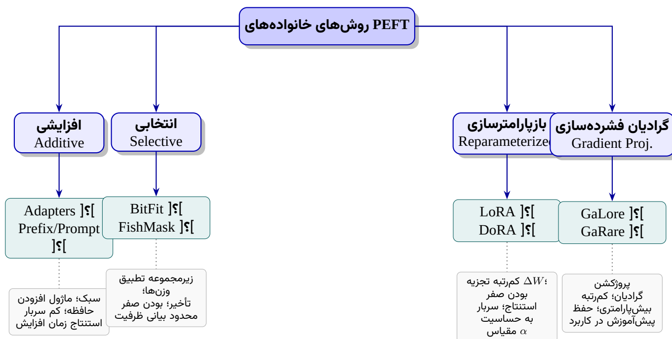
شکل ۱۰۲: رده‌بندی درختواره‌ای ساختارهای شاخص در حوزه PEFT و ویژگی‌های بنیادین هر خانواده.
