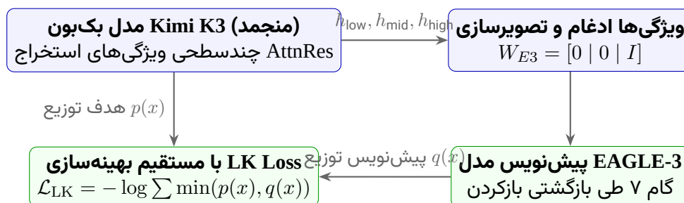
شکل ۹۶: سازوکار تقطیر مدل پیش نویس با تابع زیان LK در Kimi K3
