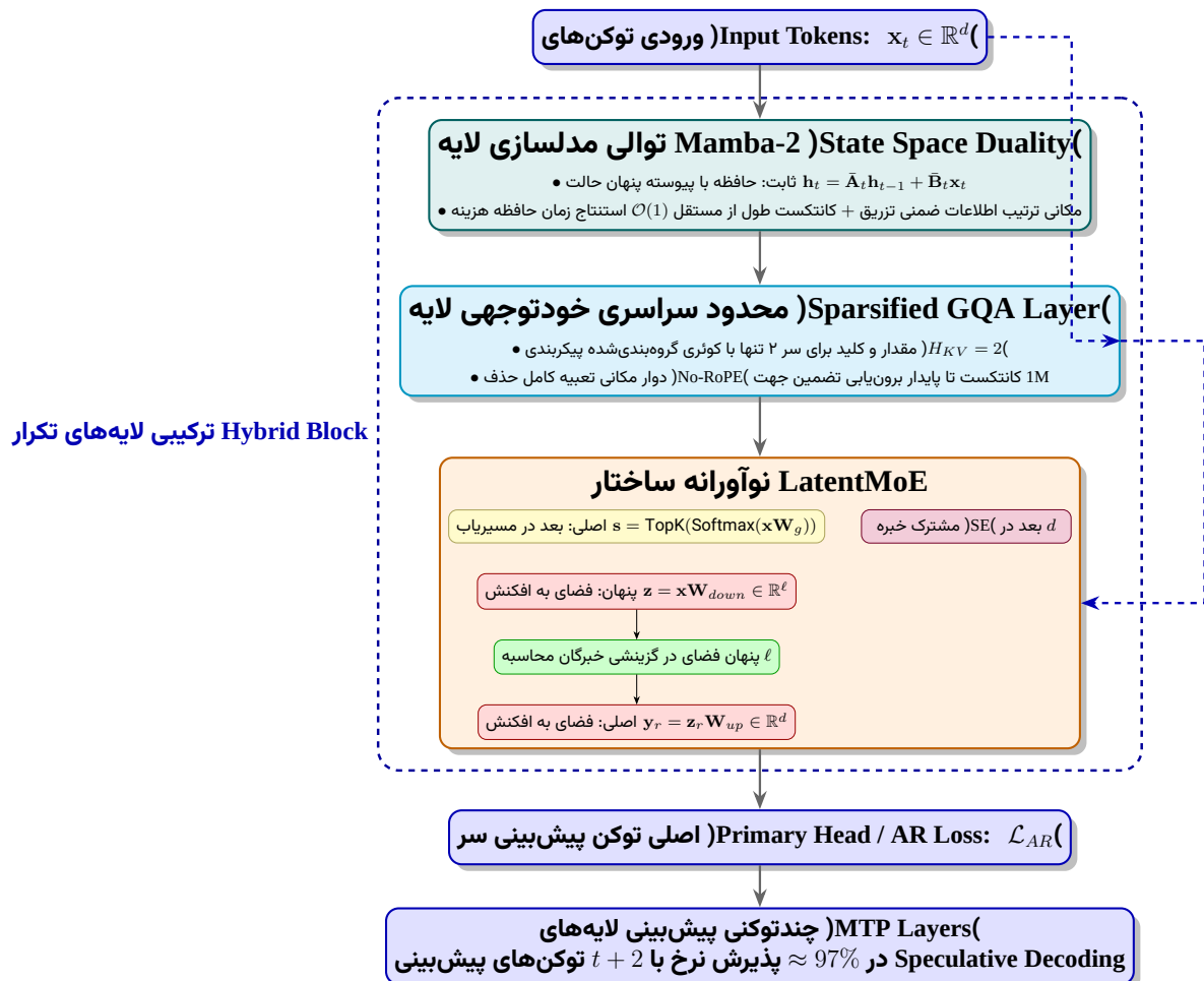
شکل ۱۹: توپولوژی جریان داده و اجزای لایه‌ای در معماری دورگه Nemotron 3 و ساختار تخصصی LatentMoE.
