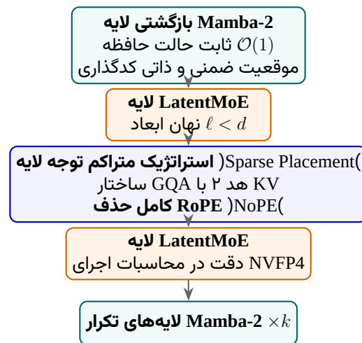
شکل ۲۹: ترکیب لایه‌های متناوب Mamba-2 و لایه‌های استراتژیک خودتوجهی فاقد RoPE در Nemotron 3.
