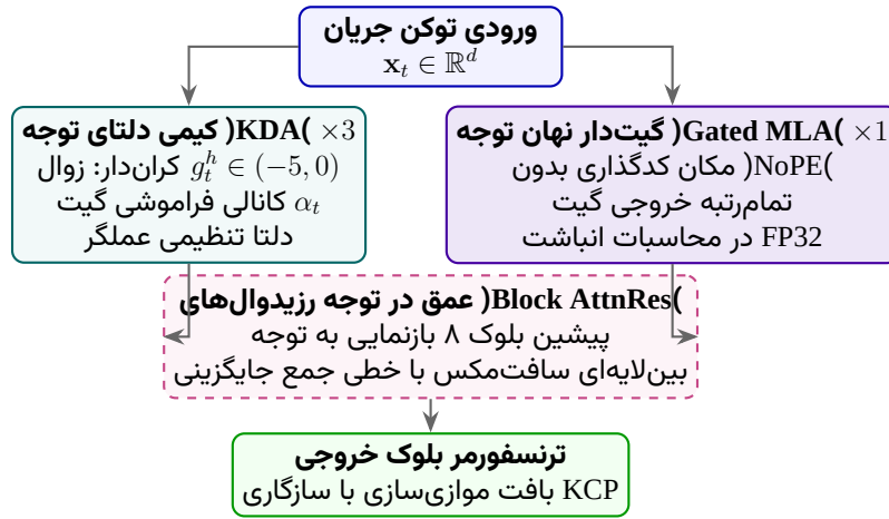
شکل ۲۵: معماری لایه توجه ترکیبی در Kimi K3: درهم‌تنیدگی KDA و Gated MLA در امتداد توالی و AttnRes در امتداد عمق.
