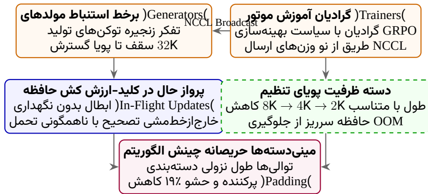
شکل ۲۶: مدیریت جریان و ماندگاری حافظه کش کلید-ارزش در خط لوله RL برخط مدل Magistral.
