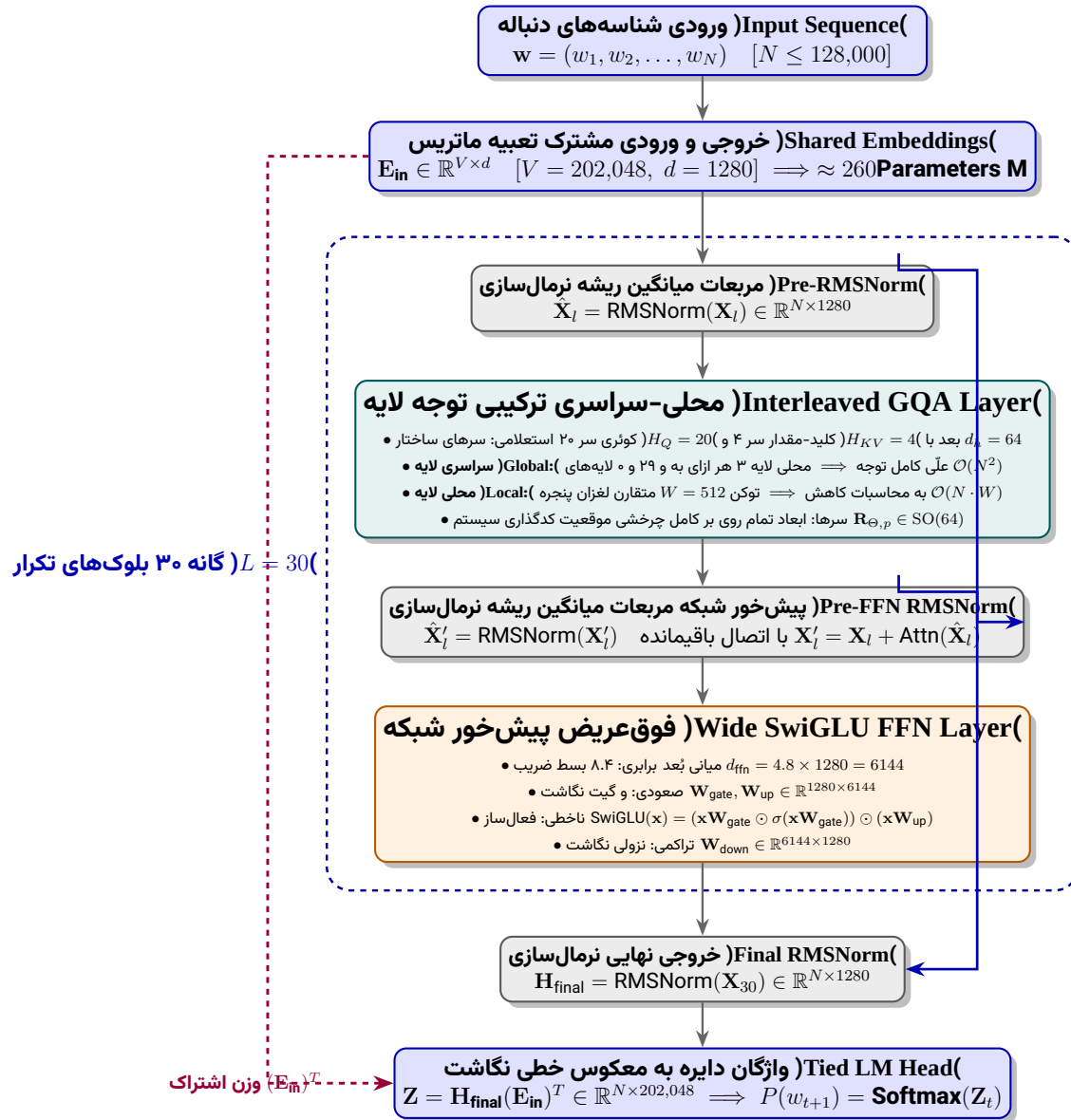
شکل ۳۷: جریان داده، تبدیل تانسورها و ساختار سلسله‌مراتبی لایه‌ها در مدل زبانی MobileLLM-Pro.
