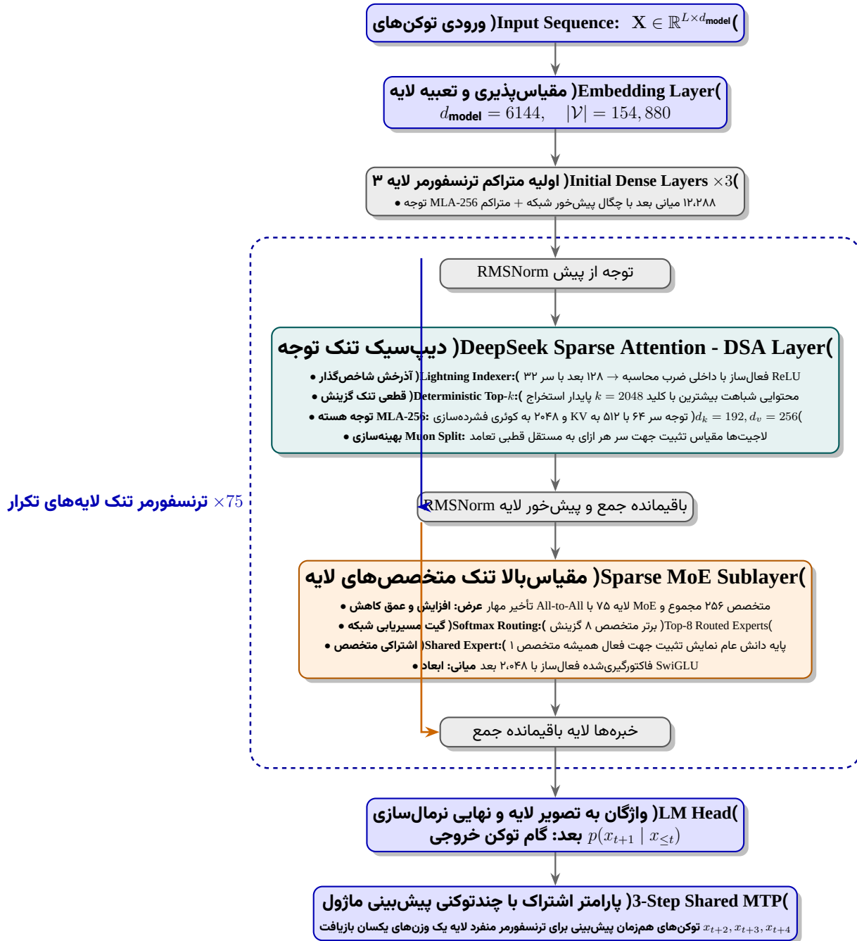
شکل ۳۳: جریان داده و تبدیل تانسورها در بلوک ترنسفورمر مدل GLM-5 شامل لایه‌های متراکم اولیه، تلفیق توجه تنک DSA با MLA-256، شبکه خبره‌های عریض و ماژول اشتراکی MTP.
