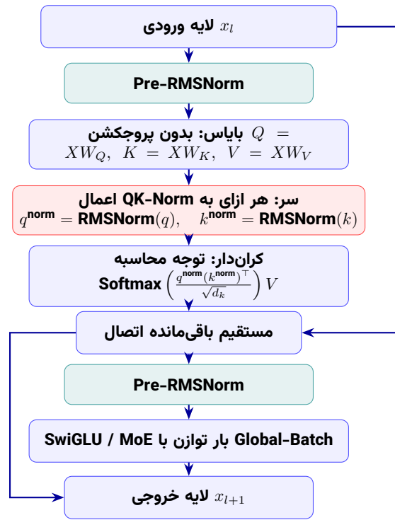
شکل ۵۱: سازوکار نرمال سازی QK-Norm و لایه های مربوطه در بلوک ترنسفورمر Qwen3
