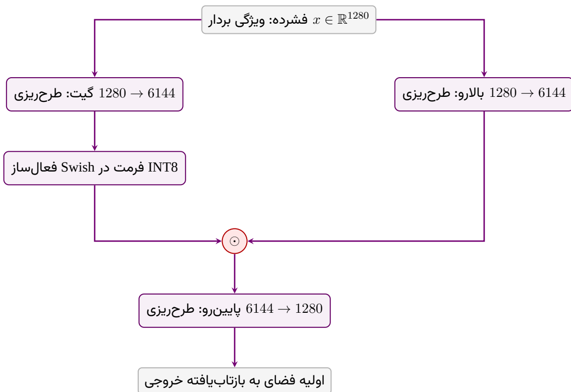
شکل ۳۷: نمودار انبساط ابعادی 4.8 \times لایه پیش‌خور در مدل بهینه‌سازی‌شده MobileLLM-Pro
