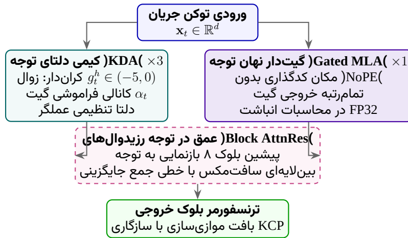
شکل ۴۵: معماری لایه توجه ترکیبی در Kimi K3: درهم‌تنیدگی KDA و Gated MLA در امتداد توالی و AttnRes در امتداد عمق.
