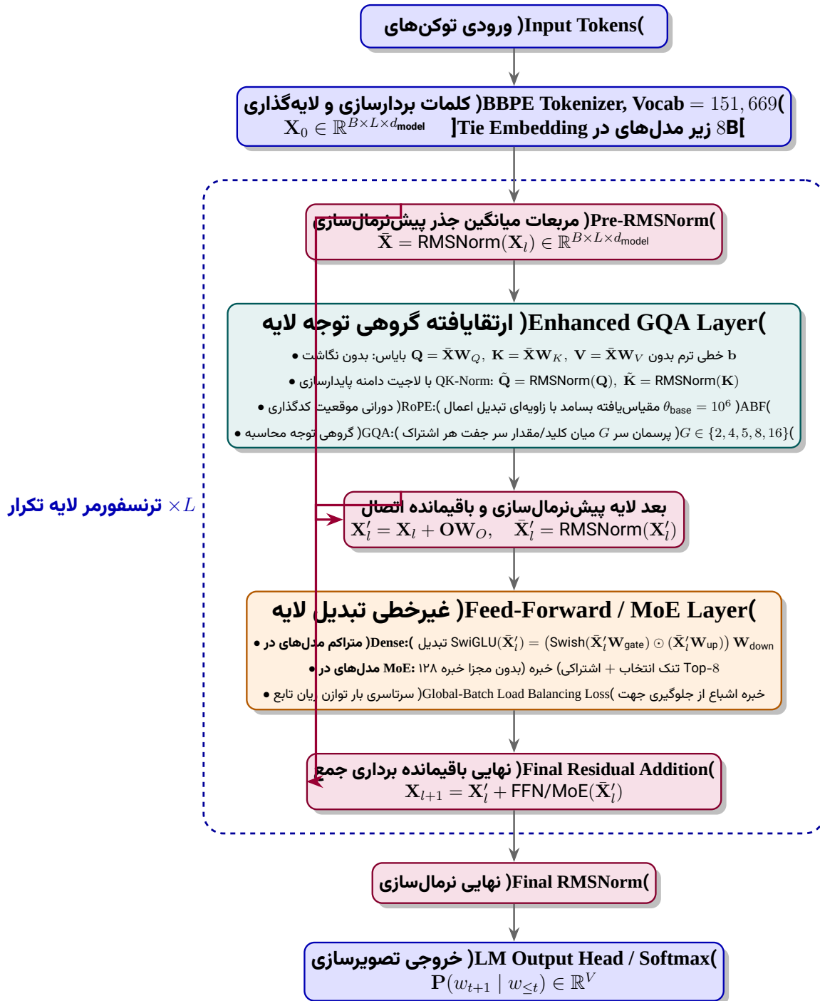
شکل ۵۹: جریان پردازش داده و تانسور در بلوک ترنسفورمر مدل Qwen3.
