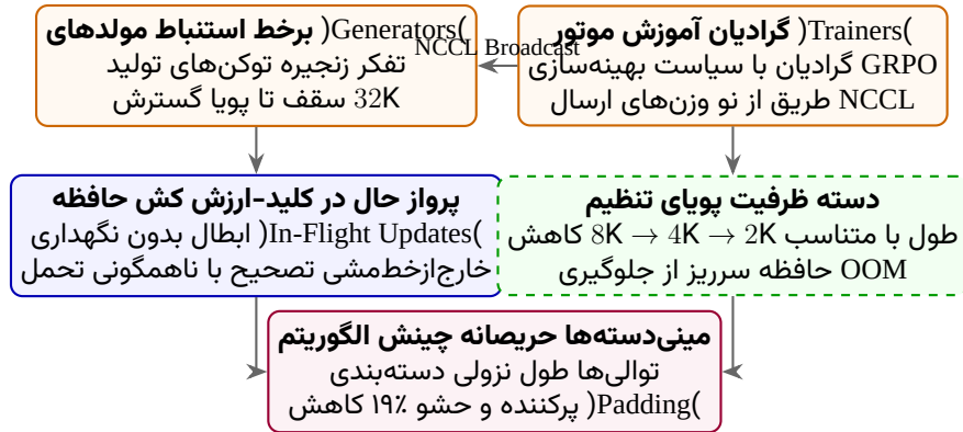
شکل ۴۶: مدیریت جریان و ماندگاری حافظه کش کلید-ارزش در خط لوله RL برخط مدل Magistral .
