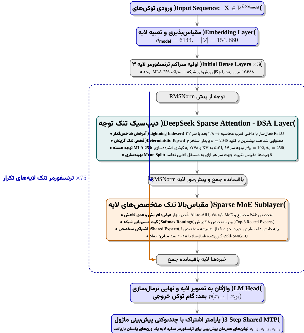
شکل ۵۳: جریان داده و تبدیل تانسورها در بلوک ترنسفورمر مدل GLM-5 شامل لایه‌های متراکم اولیه، تلفیق توجه تنک DSA با MLA-256، شبکه خبره‌های عریض و ماژول اشتراکی MTP.
