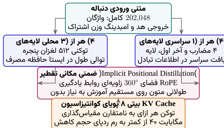
شکل ۴۸: طراحی لایه توجه هیبریدی محلی-سراسری و فرآیند تقطیر مکانی در MobileLLM-Pro.
