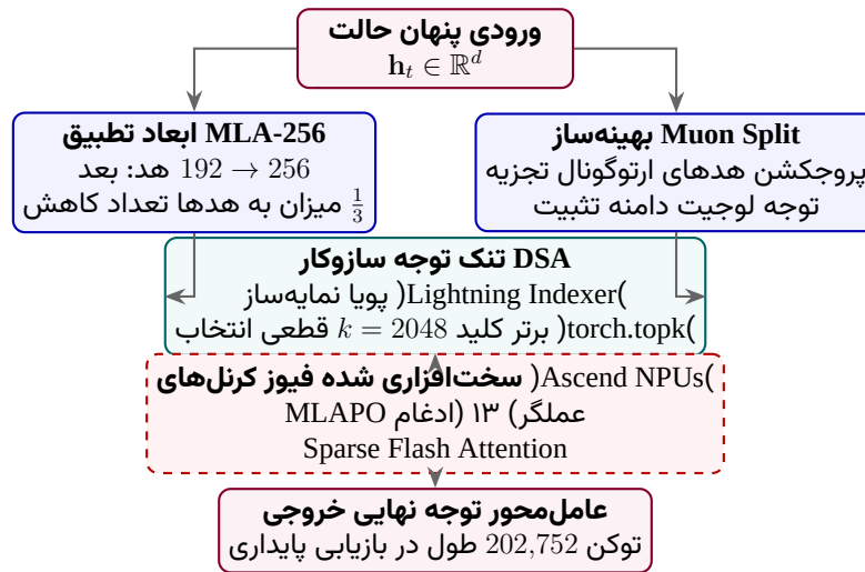
شکل ۴۴: نوآوری‌های محاسباتی و ادغام سخت‌افزاری سازوکار توجه در مدل GLM-5.
