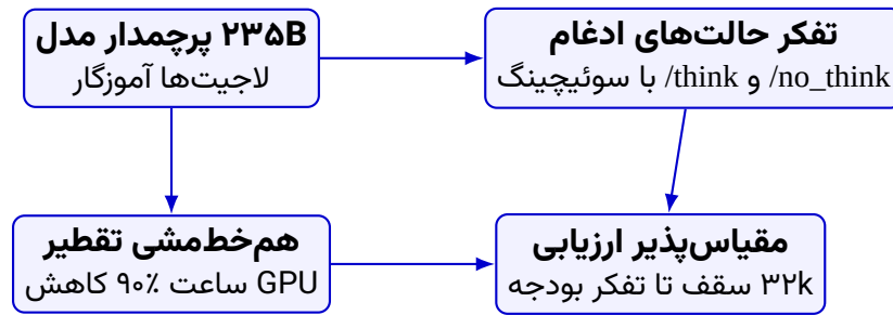
شکل ۸۹: جریان تقطیر و ارزیابی حالات پاسخ‌دهی در مدل‌های Qwen3
