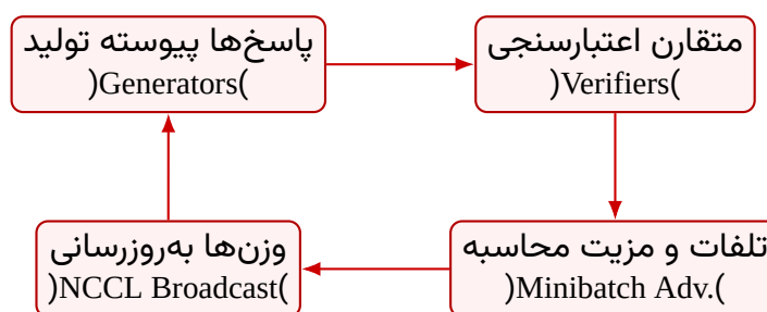
شکل ۸۶: خط لوله بازخورد بلادرنگ در ارزیابی مدل Magistral
