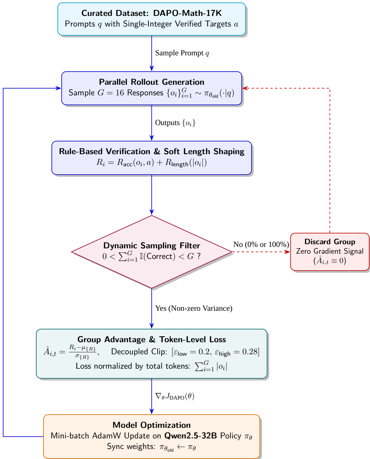
شکل ۹۴: دیاگرام جامع جریان داده، نمونه‌برداری پویا، شکل‌دهی طول و بهینه‌سازی توکن‌محور در الگوریتم DAPO.
