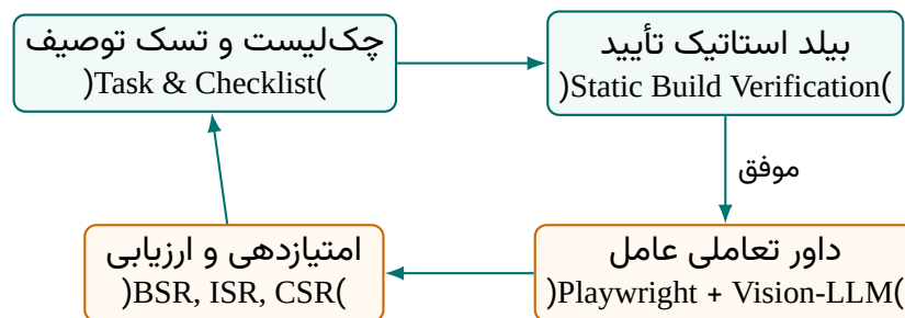
شکل ۸۴: چرخه بسته ارزیابی Agent-as-a-Judge در ارزیابی فرانت‌اند GLM-5
