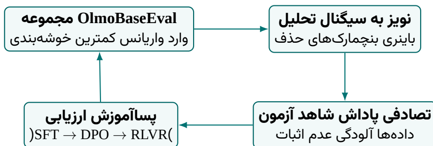
شکل ۹۰: چارچوب پایش کیفیت و عدم آلودگی داده‌ها در ارزیابی OLMo 3
