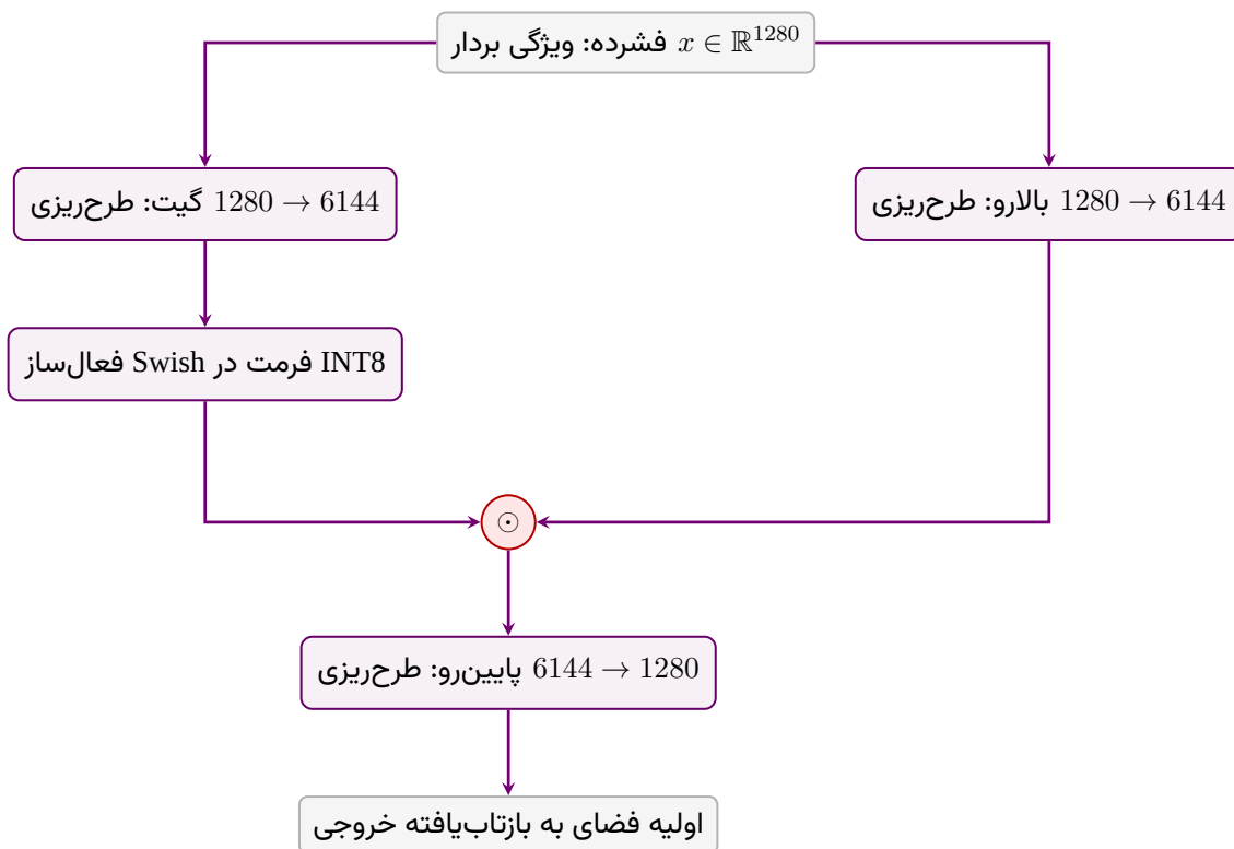
شکل ۳۷: نمودار انبساط ابعادی 4.8 \times لایه پیش‌خور در مدل بهینه‌سازی شده MobileLLM-Pro
