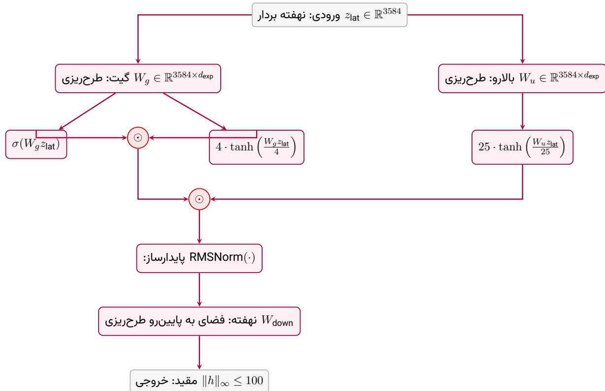
شکل ۳۴: معماری تحليلی فعال‌ساز پایدار SiTU-GLU در لایه‌های پیش‌خور مدل Kimi K3
