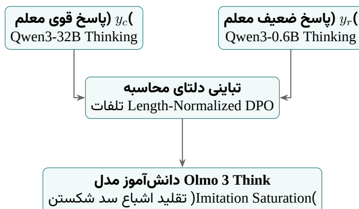
شکل ۱۰۰: سازوکار یادگیری دلتا (Delta Learning) در برابر اشباع تقلید در Olmo 3
