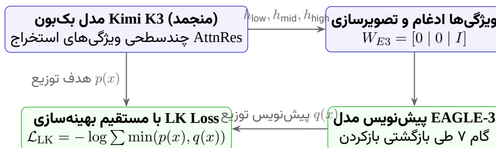
شکل ۹۵: سازوکار تقطیر مدل پیش‌نویس با تابع زیان LK در Kimi K3
