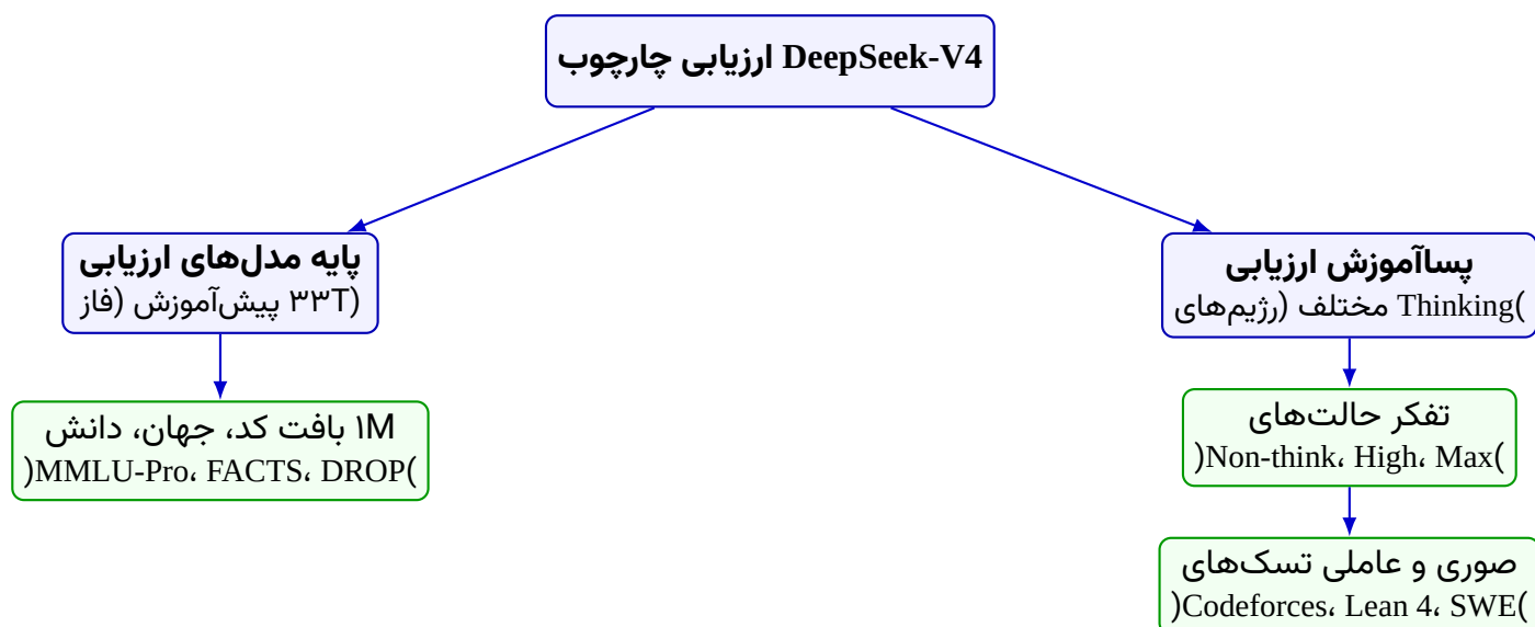
شکل ۱۰۱: جریان ساختار ارزیابی چندبعدی در مدل DeepSeek-V4
