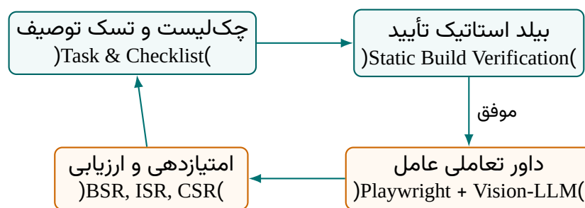
شکل ۱۰۲: چرخه بسته ارزیابی Agent-as-a-Judge در ارزیابی فرانت‌اند GLM-5
