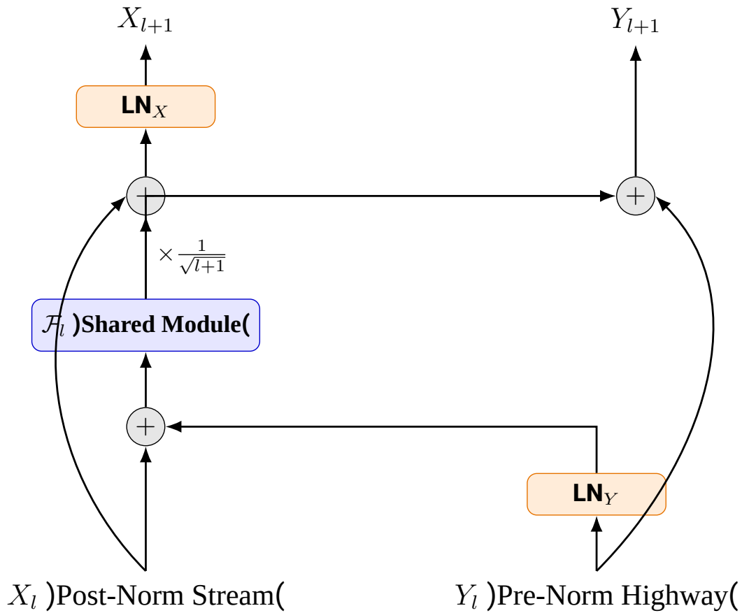
شکل ۴۳: معماری دوجریانی SiameseNorm [۳۸۵] با جداسازی بزرگراه خطی و جریان فشرده.
