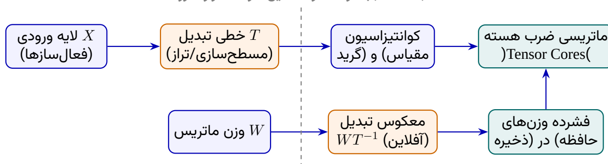
شکل ۸۳: جریان پردازش داده در خط لوله کوانتیزاسیون مدرن مدل‌های زبانی بزرگ.
