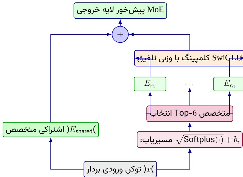
شکل ۲۳: ساختار بلوک پیش‌خور MoE در مدل DeepSeek-V4 همراه با مخصص اشتراکی و گیتینگ رادیکال سافت‌پلاس.
