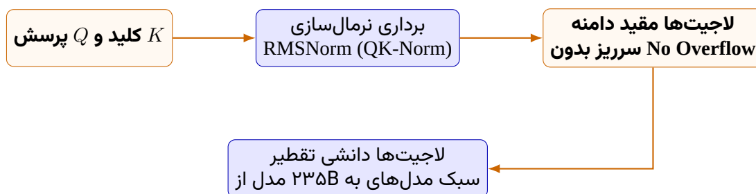
شکل ۹۱: پایدارسازی دامنه لاجیت با QK-Norm و انتقال تقطیری در Qwen3
