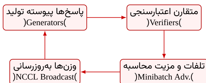
شکل ۱۰۴: خط لوله بازخورد بلادرنگ در ارزیابی مدل Magistral
