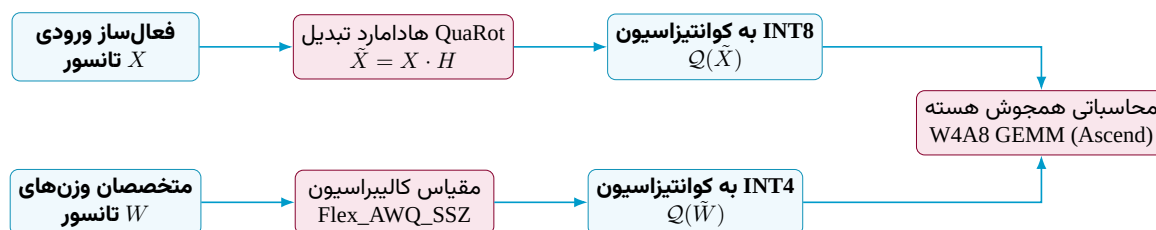
شکل ۸۶: سامانه کوانتیزاسیون مختلط W4A8 با تبدیل هادامارد در GLM-5
