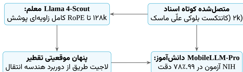
شکل ۹۸: انتقال فضای زاویه‌ای RoPE از طریق تقطیر موقعیتی پنهان در MobileLLM-Pro
