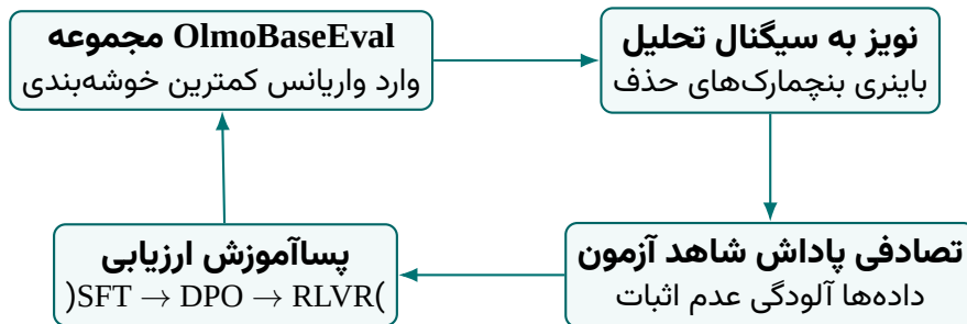
شکل ۱۰۸: چارچوب پایش کیفیت و عدم آلودگی داده‌ها در ارزیابی OLMo 3
