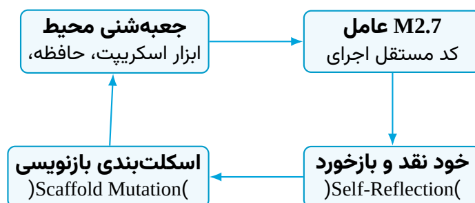
شکل ۱۰۵: چرخه بازگشتی خودتکاملی و ارزیابی در مدل MiniMax-M2.7
