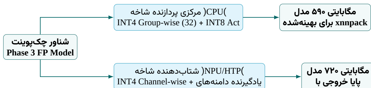
شکل ۹۰: خط لوله دوگانه کوانتیزاسیون ۴ بیتی و خود-تقطیر دانشی در MobileLLM-Pro
