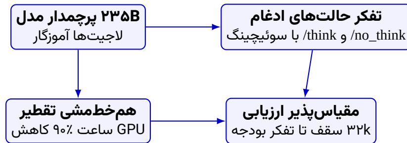
شکل ۱۰۷: جریان تقطیر و ارزیابی حالات پاسخ‌دهی در مدل‌های Qwen3
