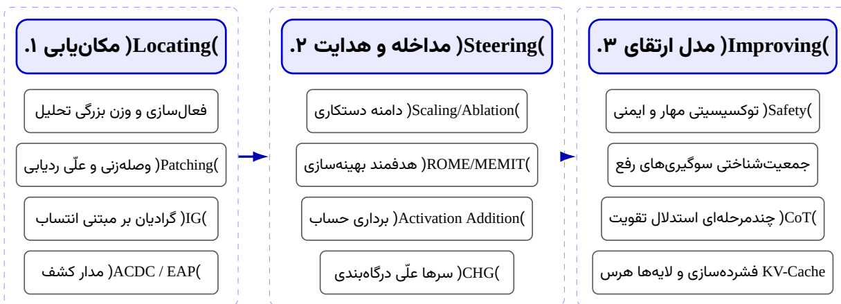
شکل ۵۴: خط لوله جامع تفسیرپذیری مکانیکی کنش‌پذیر (Locate, Steer, and Improve Pipeline) [۴۱۵].
