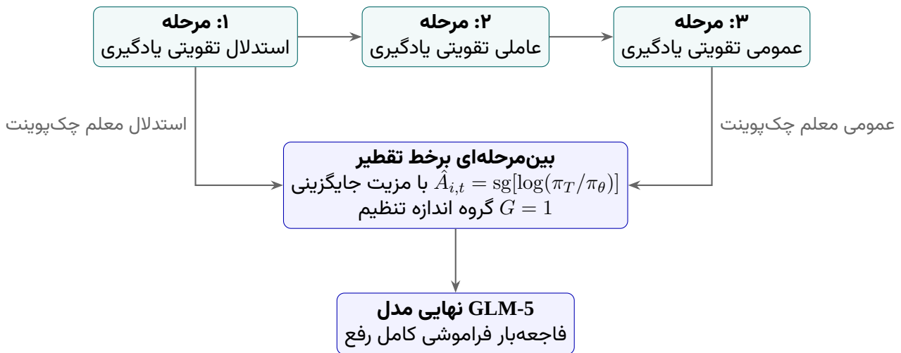
شکل ۹۴: خط لوله تقطیر برخط بین مرحله‌ای در GLM-5 برای بازیابی مهارت‌ها
