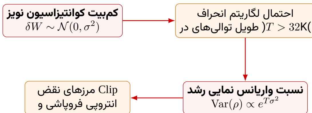
شکل ۸۸: مدل سازی انتشار خطای کوانتیزاسیون در توالی های بلند استدلالی در تحلیل مدل Magistral
