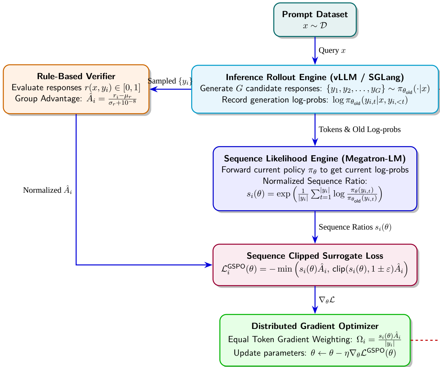
شکل ۱۱: دیاگرام جامع معماری خط لوله آموزش، محاسبه نسبت اهمیت توالی با نرمال‌سازی طولی و به‌روزرسانی گرادین همگن در الگوریتم GSPO.
