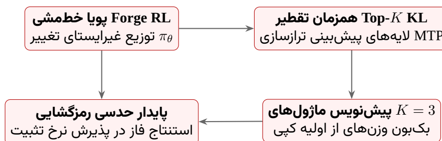
شکل ۹۷: تقطیر همزمان لایه های MTP با استفاده از Top-K KL در MiniMax-M2
