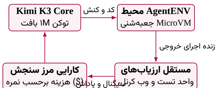
شکل ۱۰۳: چارچوب ارزیابی جعبه‌شنی و سنجش کارایی هزینه در Kimi K3
