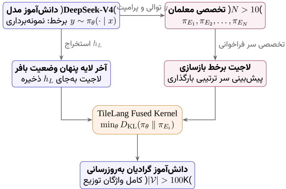
شکل ۹۳: سازوکار تقطیر برخط چندمعلمی با بازسازی بلادرنگ لاجیت در DeepSeek-V4
