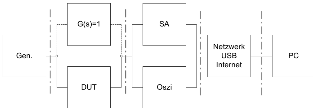
Abb. 1: Schematischer Aufbau des Versuchs[oA22]
