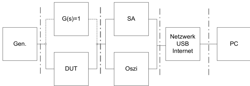
Abb. 1: Schematischer Aufbau des VersuchsoA:2022:bk
