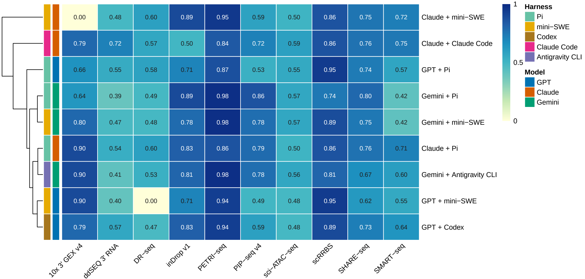
Task 3 molecular-transition F1
