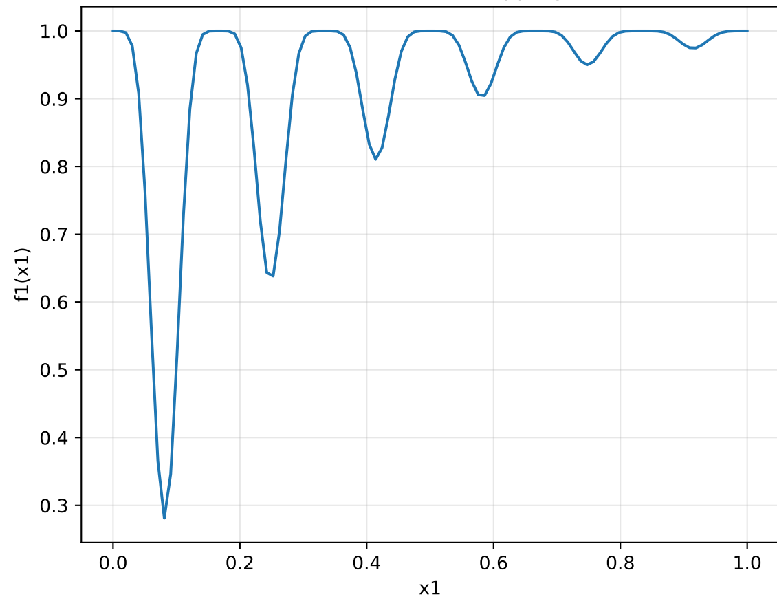
Non-uniform f1 mapping
