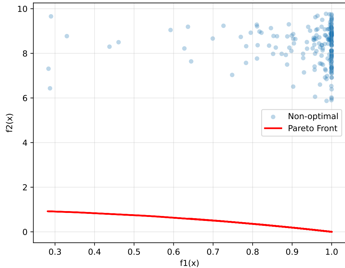
ZDT6: Non-Uniform Density
