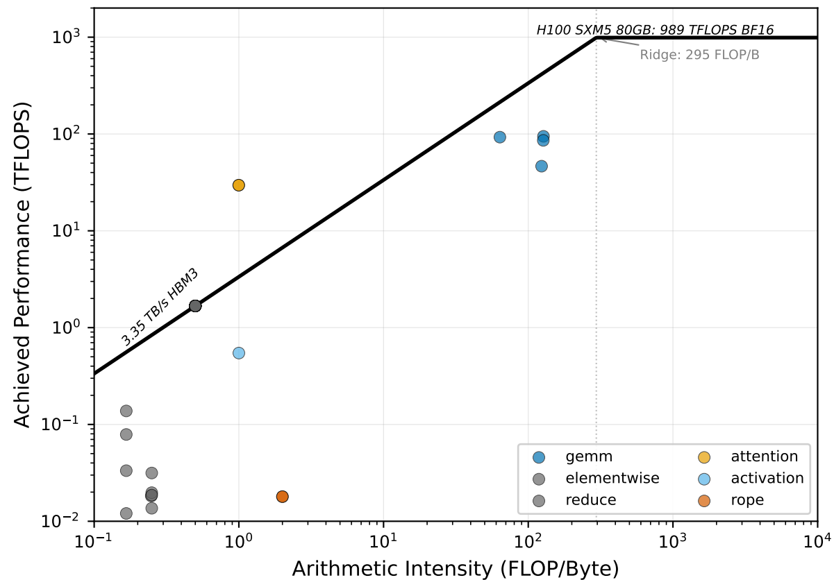
Llama-3.1-70B-Instruct — decode (BS=32)
