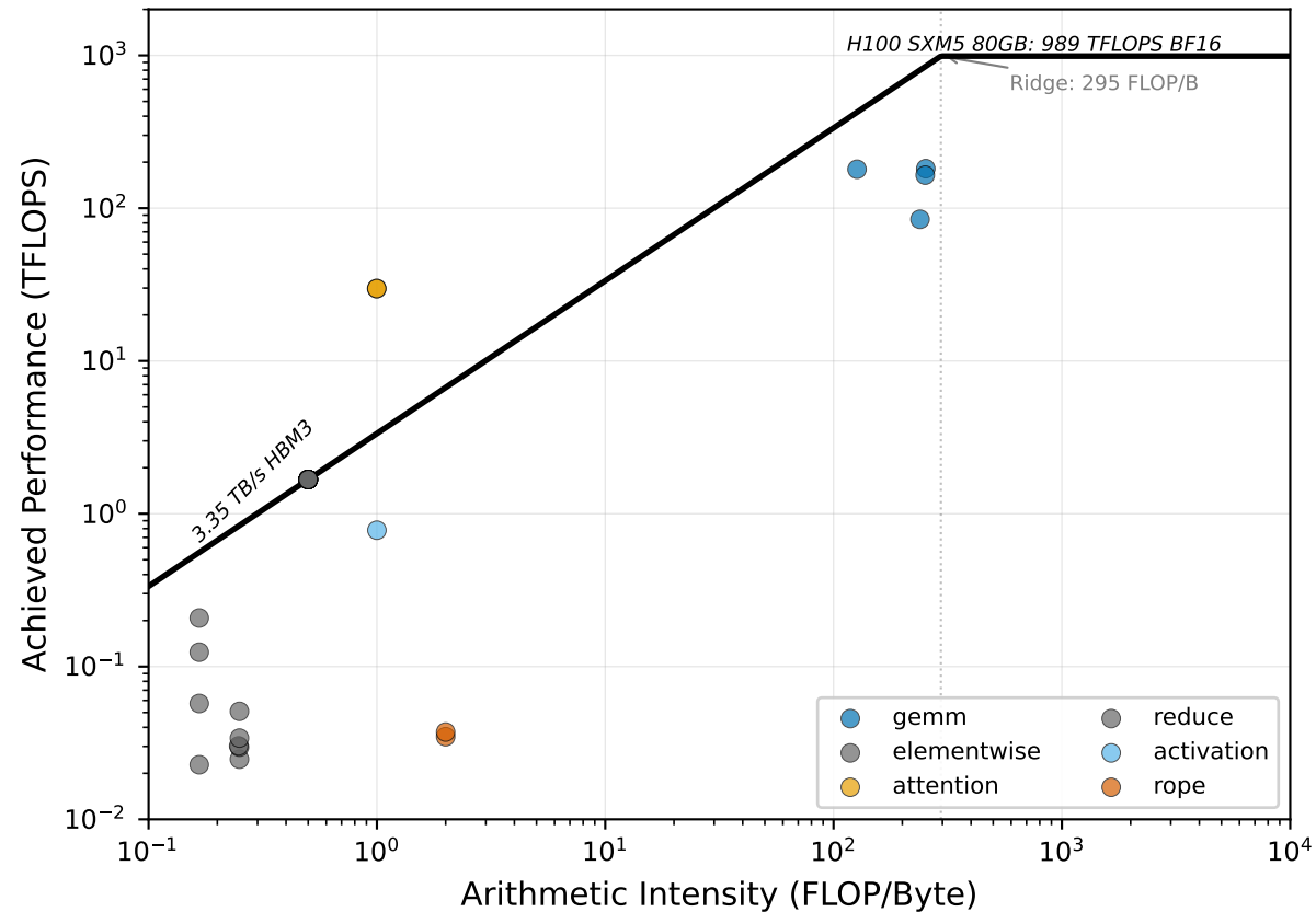
Llama-3.1-70B-Instruct — decode (BS=64)
