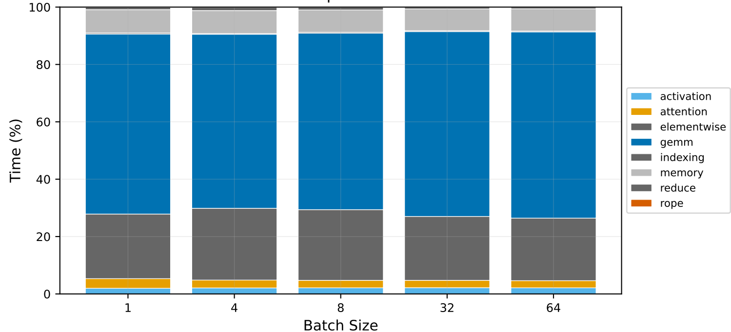
Llama-3.1-70B-Instruct — prefill Kernel Time Breakdown
