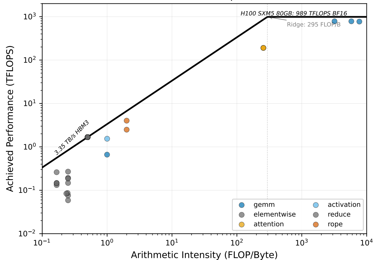
Llama-3.1-8B-Instruct — prefill (BS=64)
