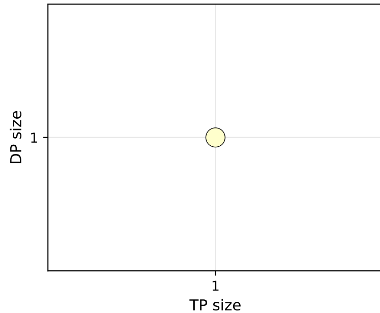
1 GPUs
