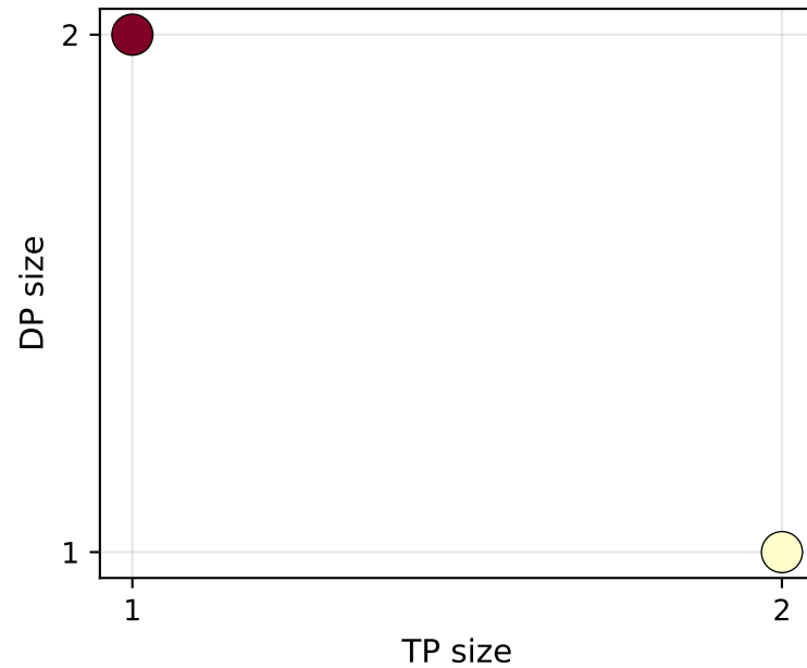
2 GPUs
