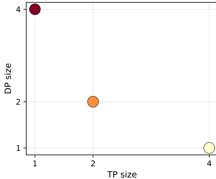
4 GPUs
