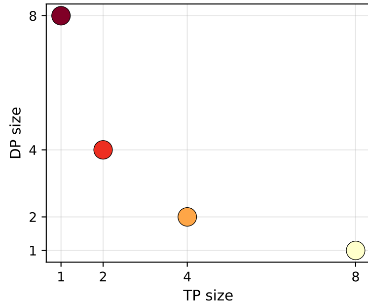
8 GPUs
