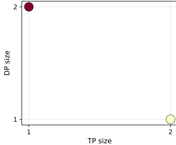
2 GPUs
