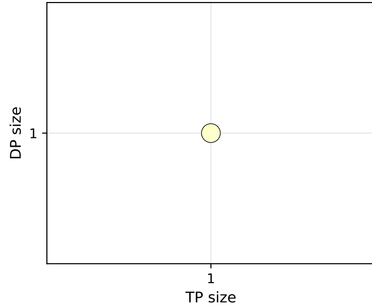
1 GPUs
