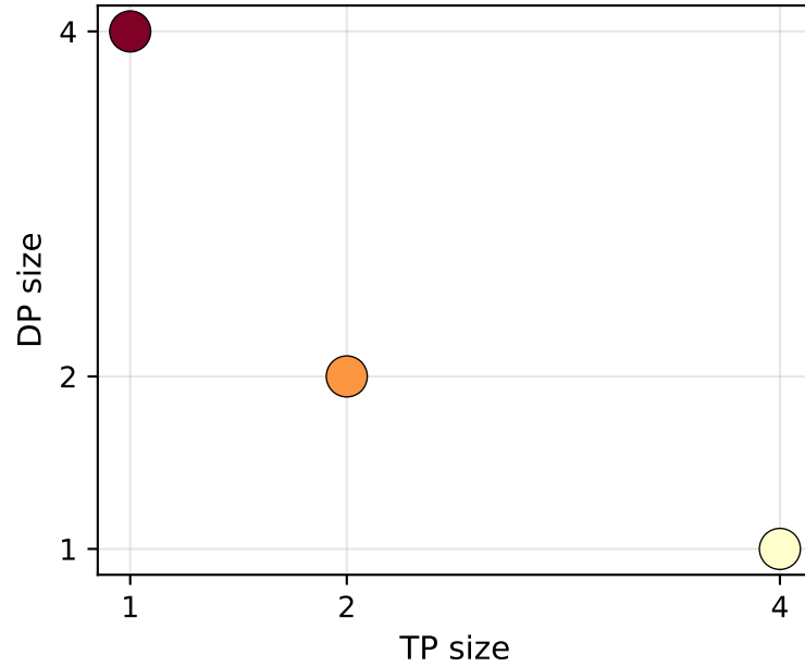
4 GPUs
