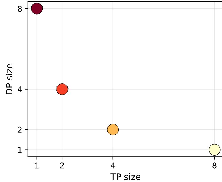
8 GPUs
