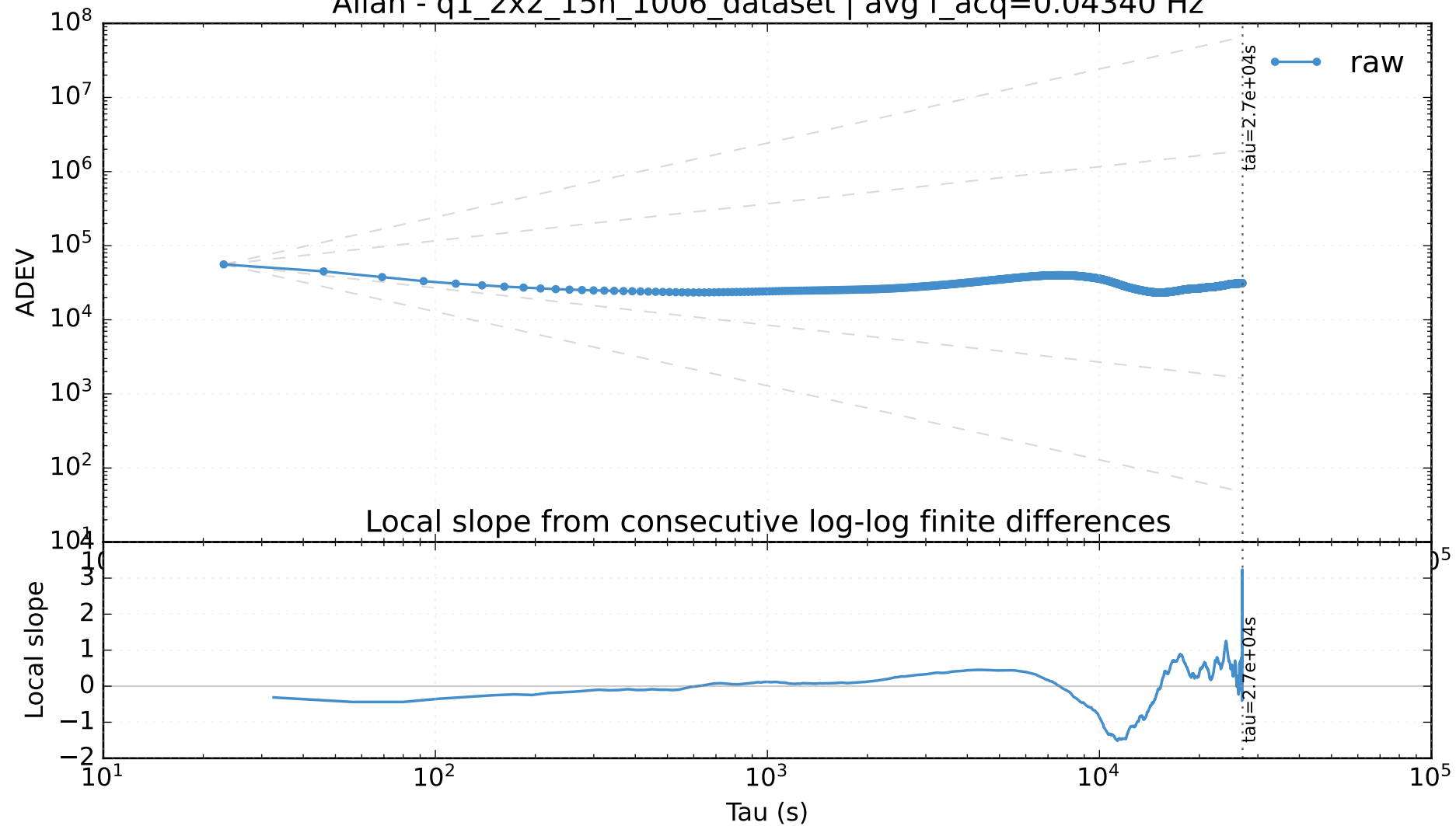
Allan - q1_2x2_15h_1006_dataset | avg f_acq=0.04340 Hz
