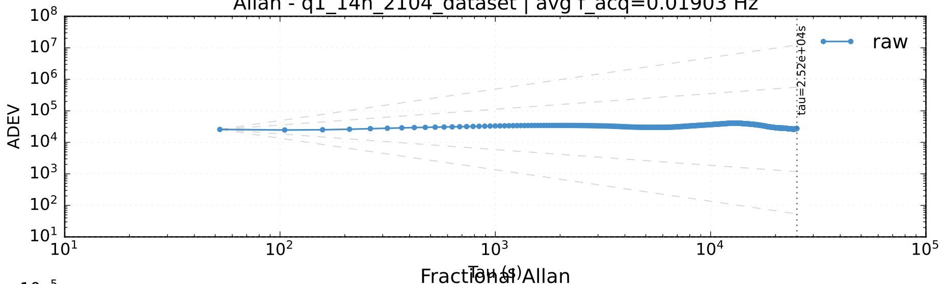
Allan - q1_14h_2104_dataset | avg f_acq=0.01903 Hz
