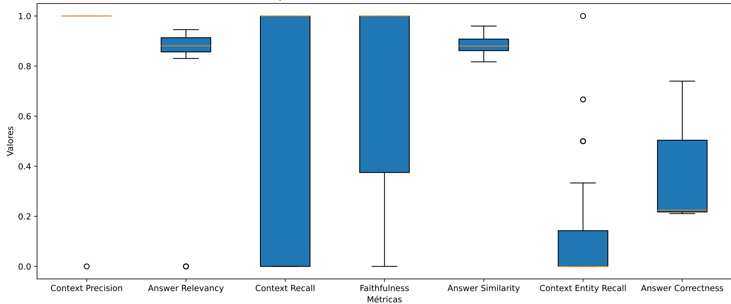
Distribuição das Métricas (RAGAS) no modelo mistral:latest
