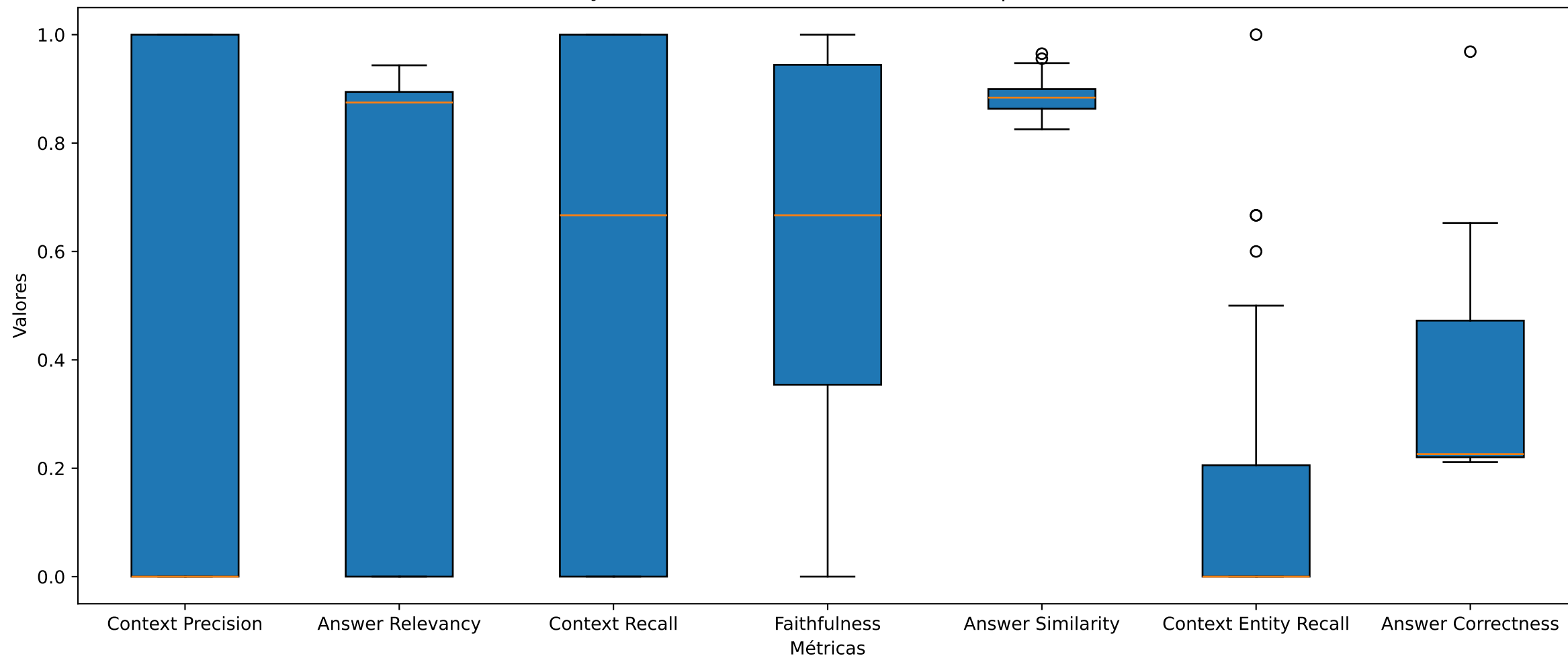
Distribuição das Métricas (RAGAS) no modelo qwen2.5:latest
