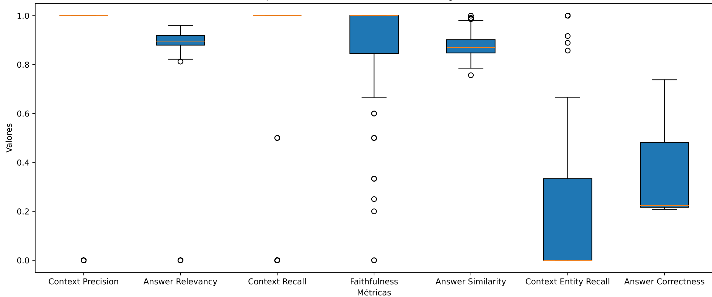
Distribuição das Métricas (RAGAS) no modelo gemma2:latest
