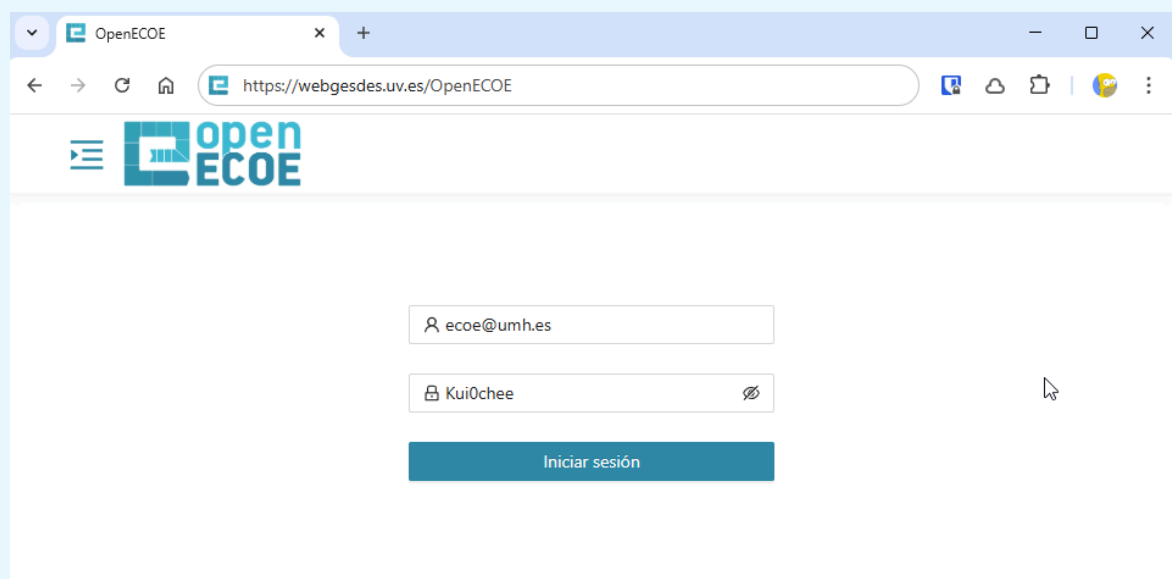
Figura 2: Login
