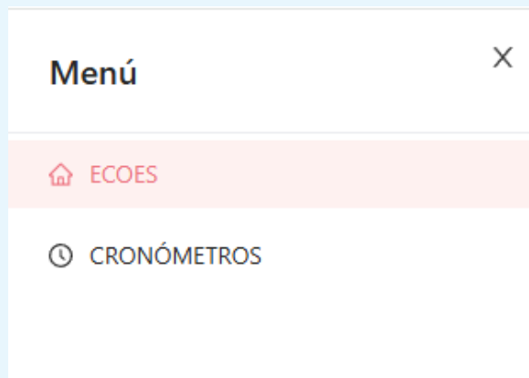
Figura 39: Menú lateral
