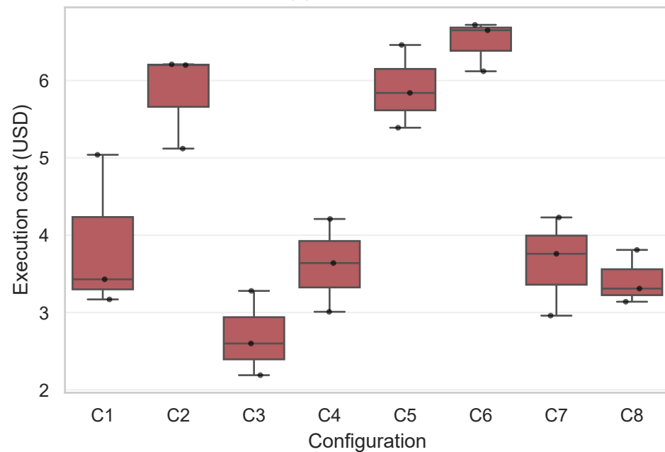
(d) Execution cost
